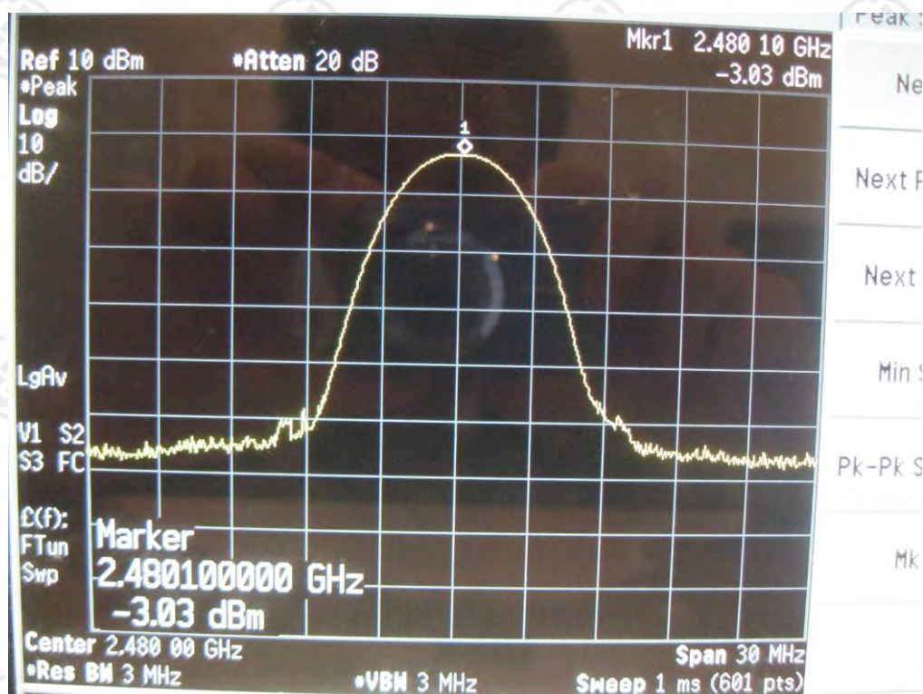
2480MHz
