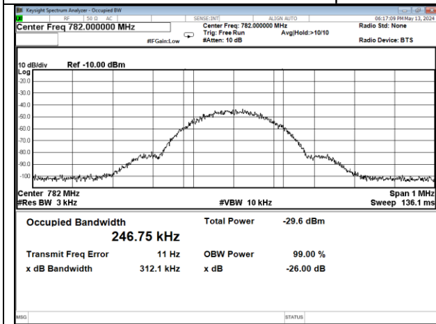
GSM-Upper 700MHz band UL input
