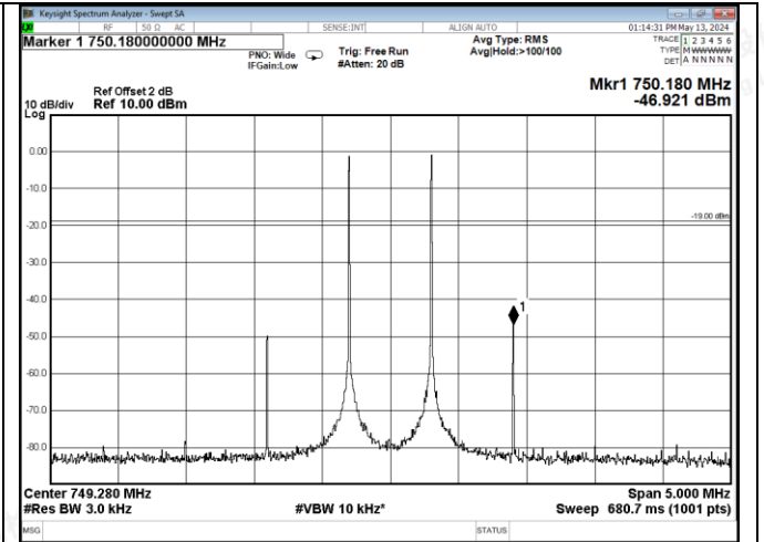
Upper 700MHz band AGC+10dB, DL
