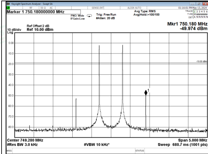
Upper 700MHz band Pre AGC, DL
