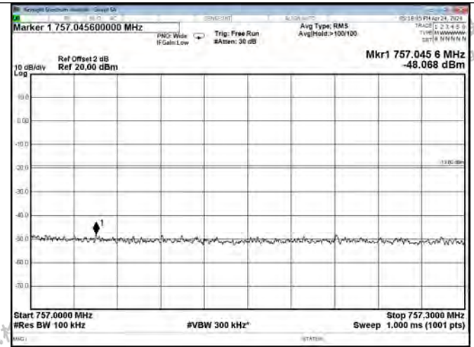
Upper 700 Band DL-LTE Right Side AGC+10dB
