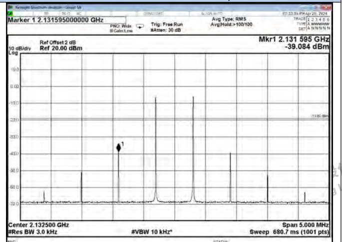
AWS Band AGC+10dB, DL
