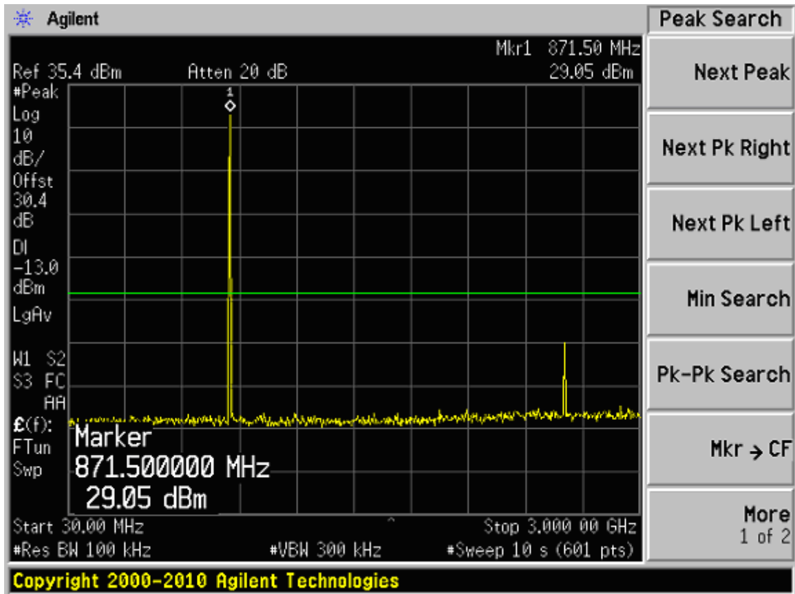
(30MHz – 3GHz)
