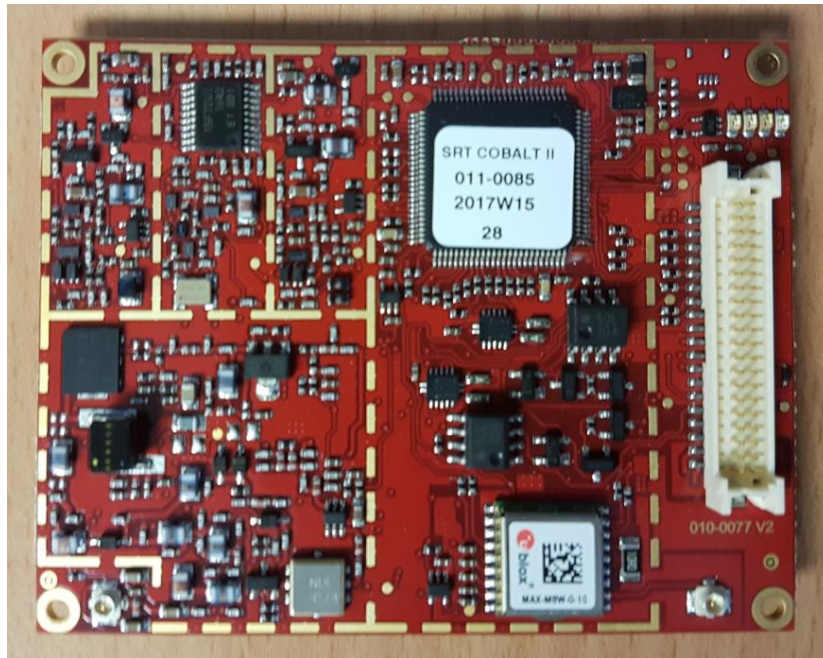
1. PCB Top
