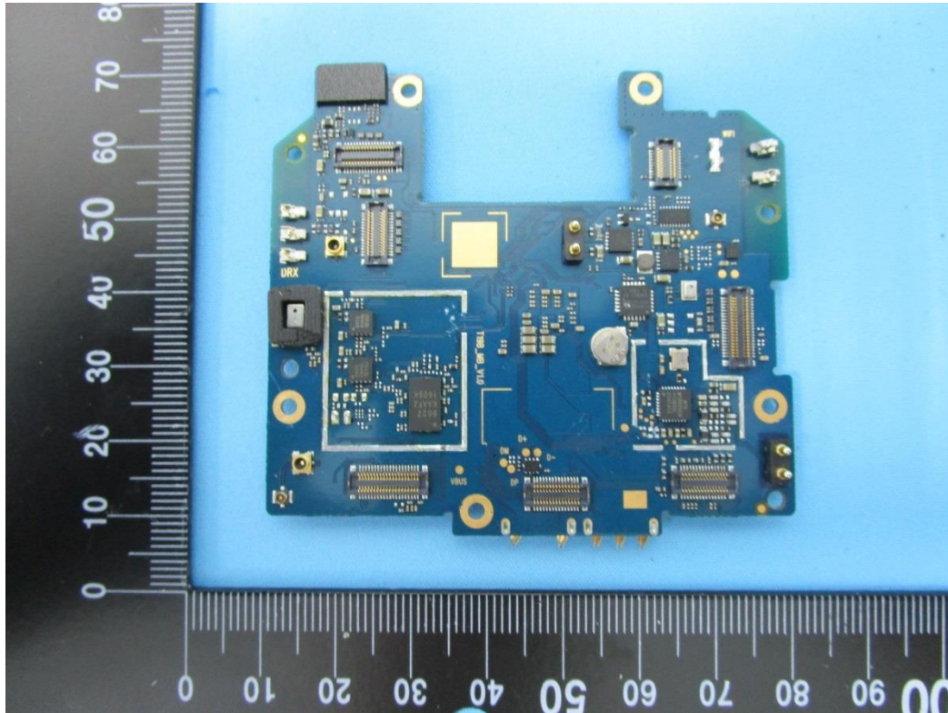
(6) EUT Photo
