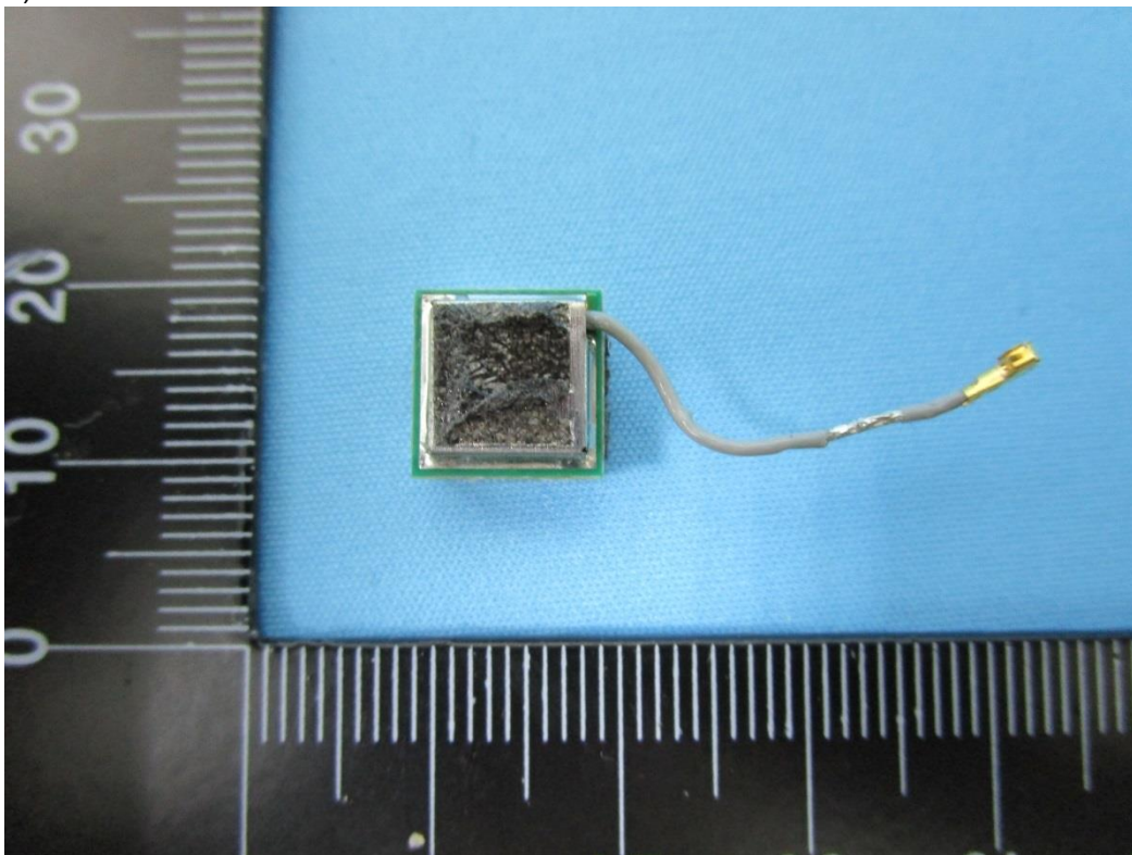
(20) EUT Photo
