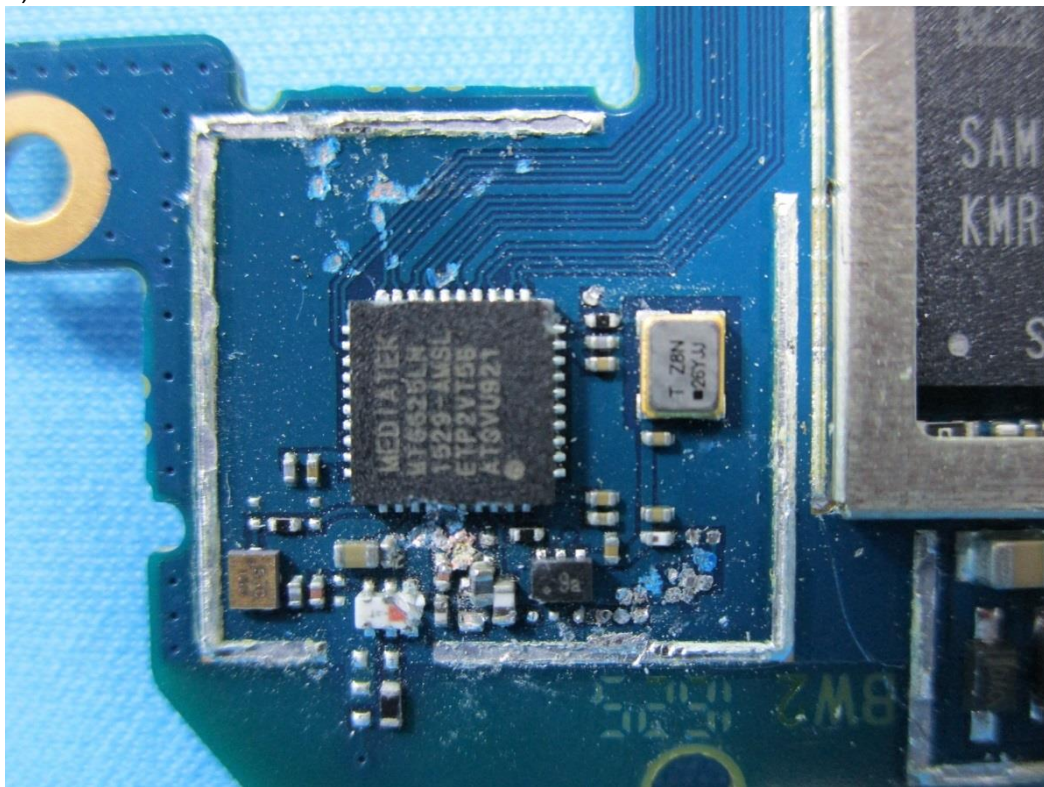
(10) EUT Photo
