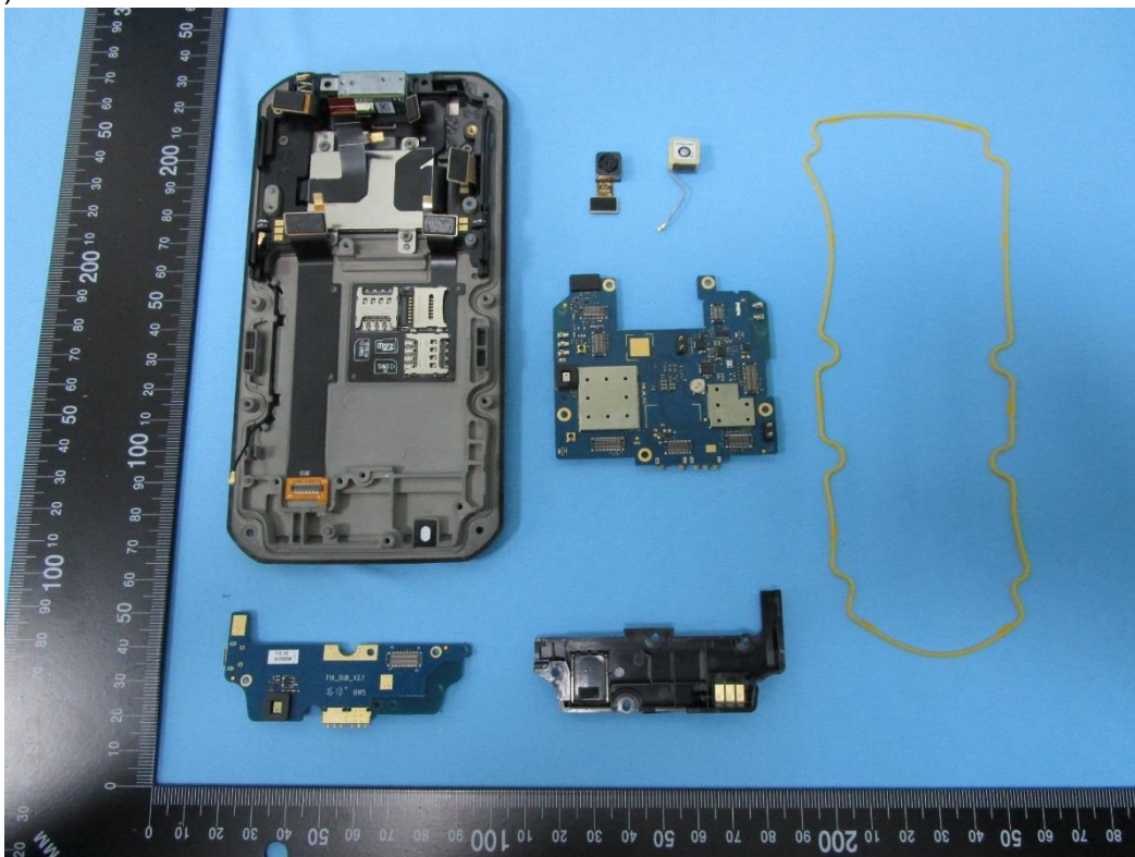
(2) EUT Photo
