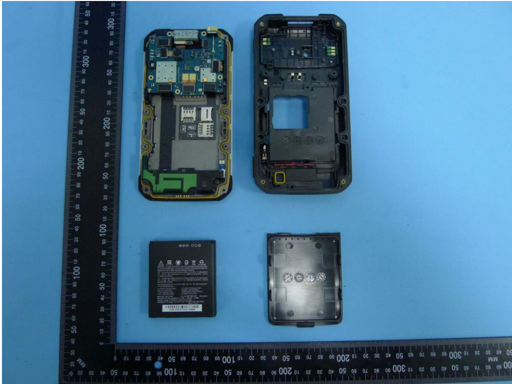
(2) EUT Photo
