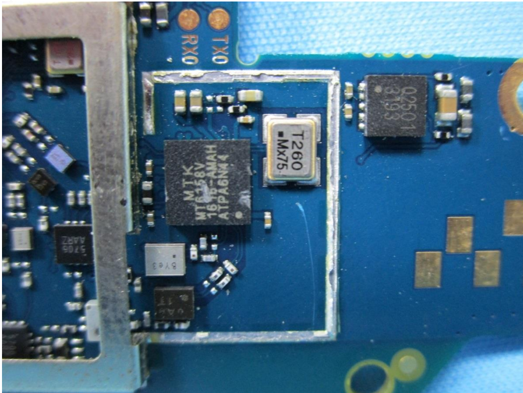
(14) EUT Photo
