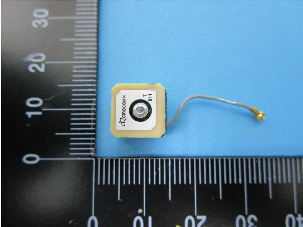
(20) EUT Photo
