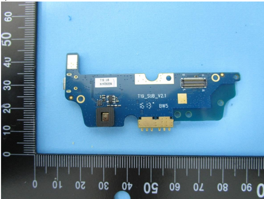
(14) EUT Photo
