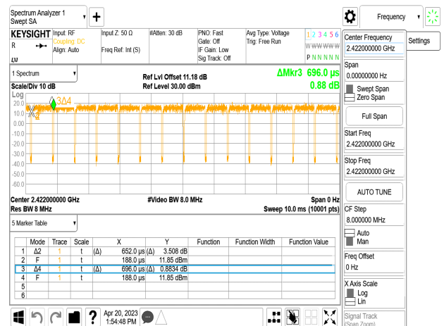
802.11ac_40MHz_Chain0_2422MHz
