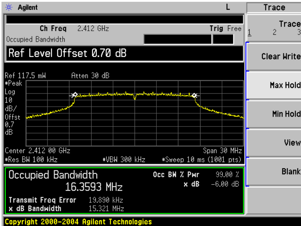
- 802.11g 1CH -
