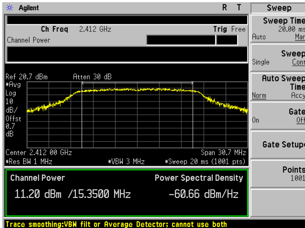
- 802.11n 1CH (Average Power)-
