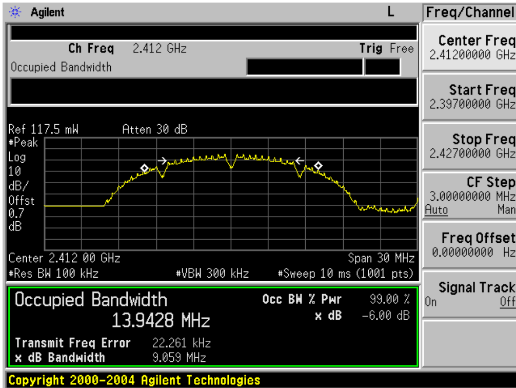
- 802.11b 1CH -
