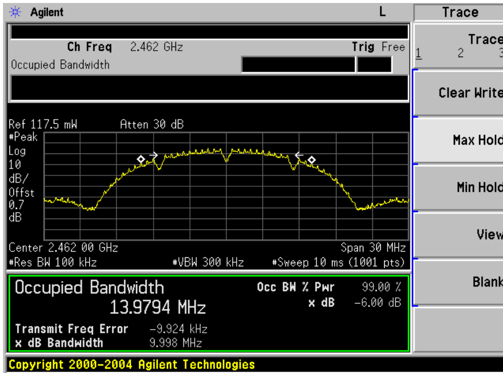
- 802.11b 11CH -
