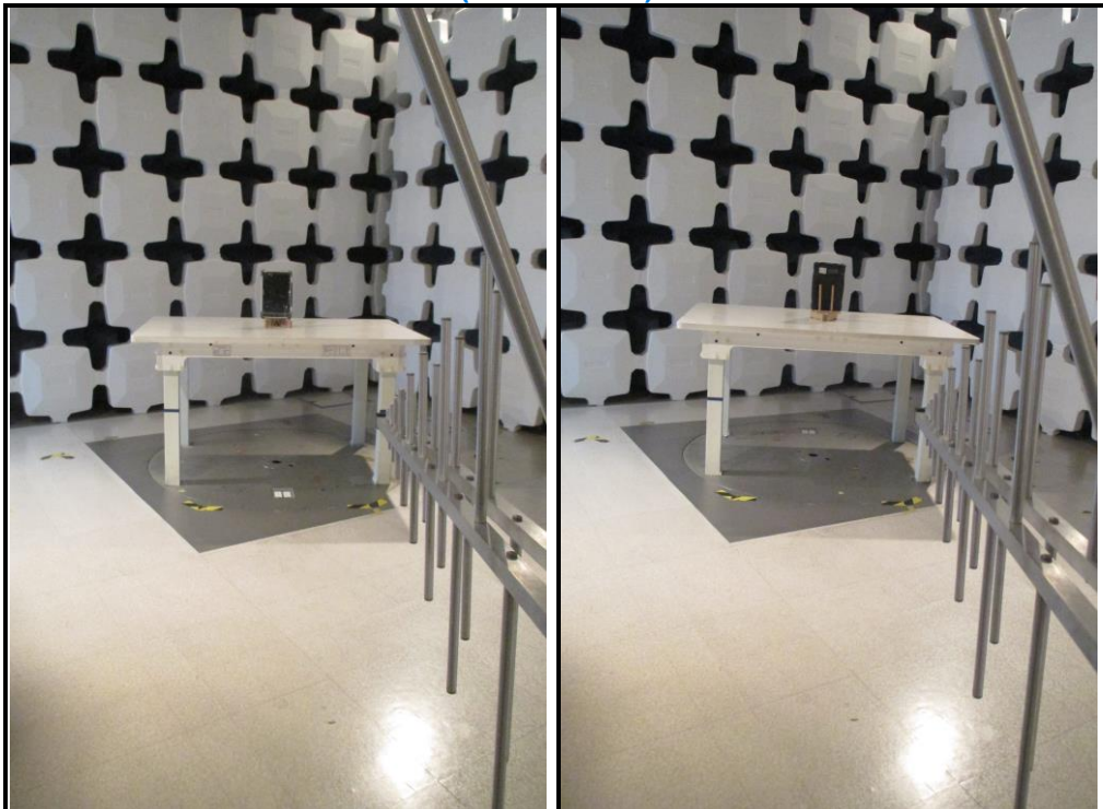
ERP POWER TEST (WCDMALTE)
