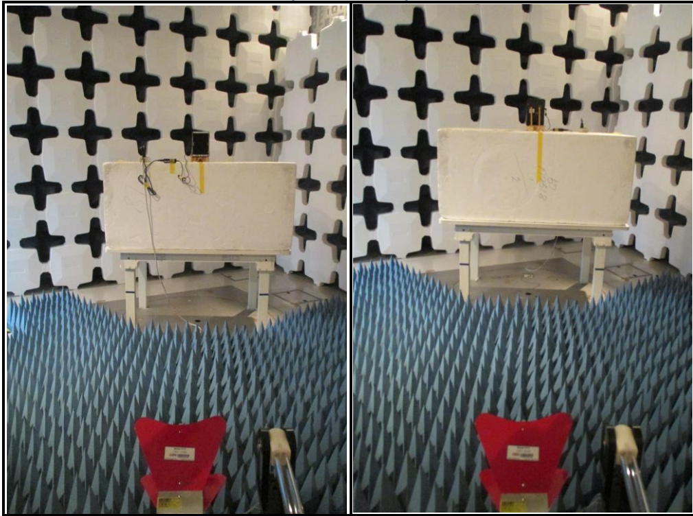
ERP POWER TEST (WCDMALTE)
