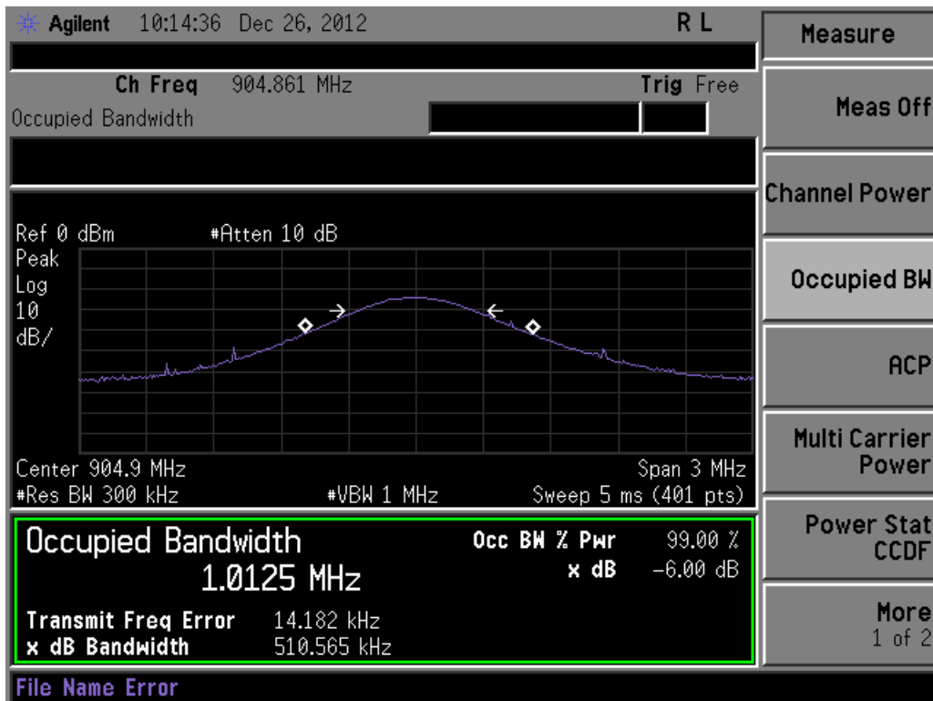
Plot - TX-904.861MHz-99% BW
