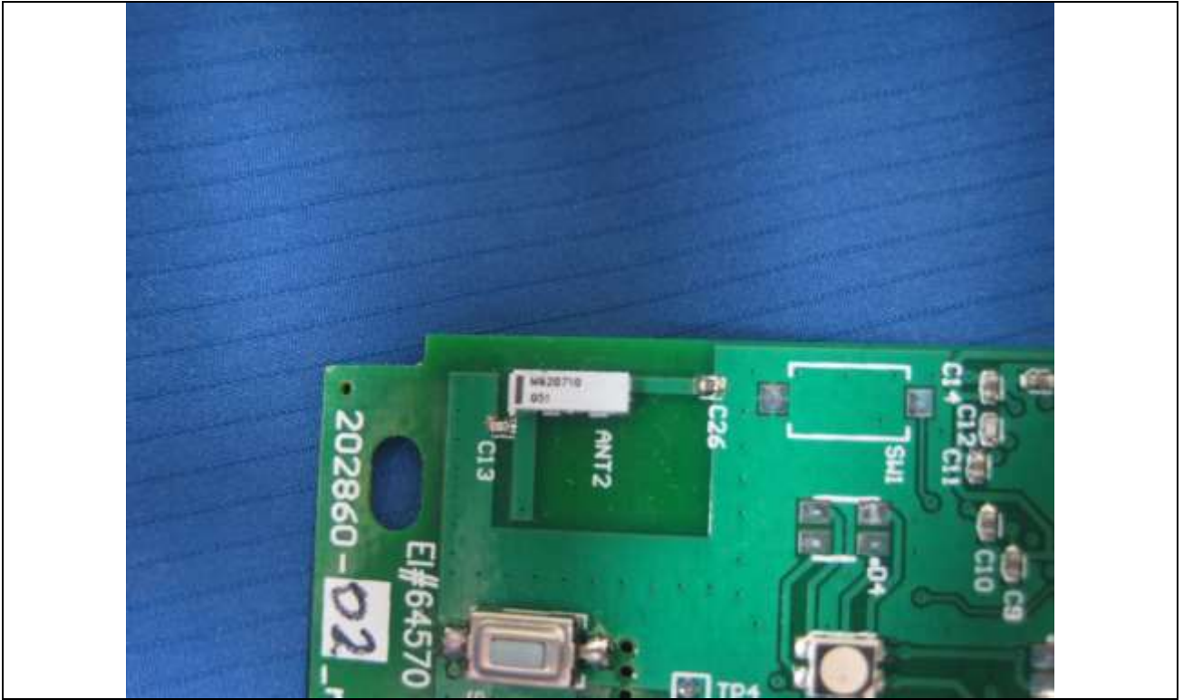
EUT - Antenna
