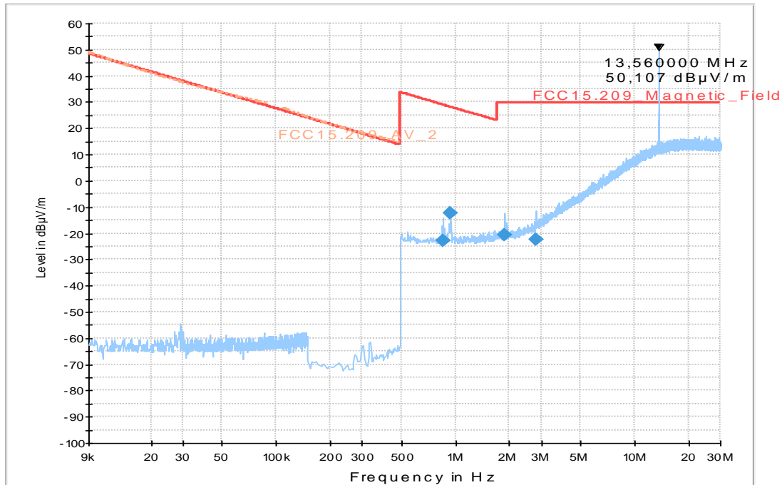
FCC 15.209_magn hor+vert
