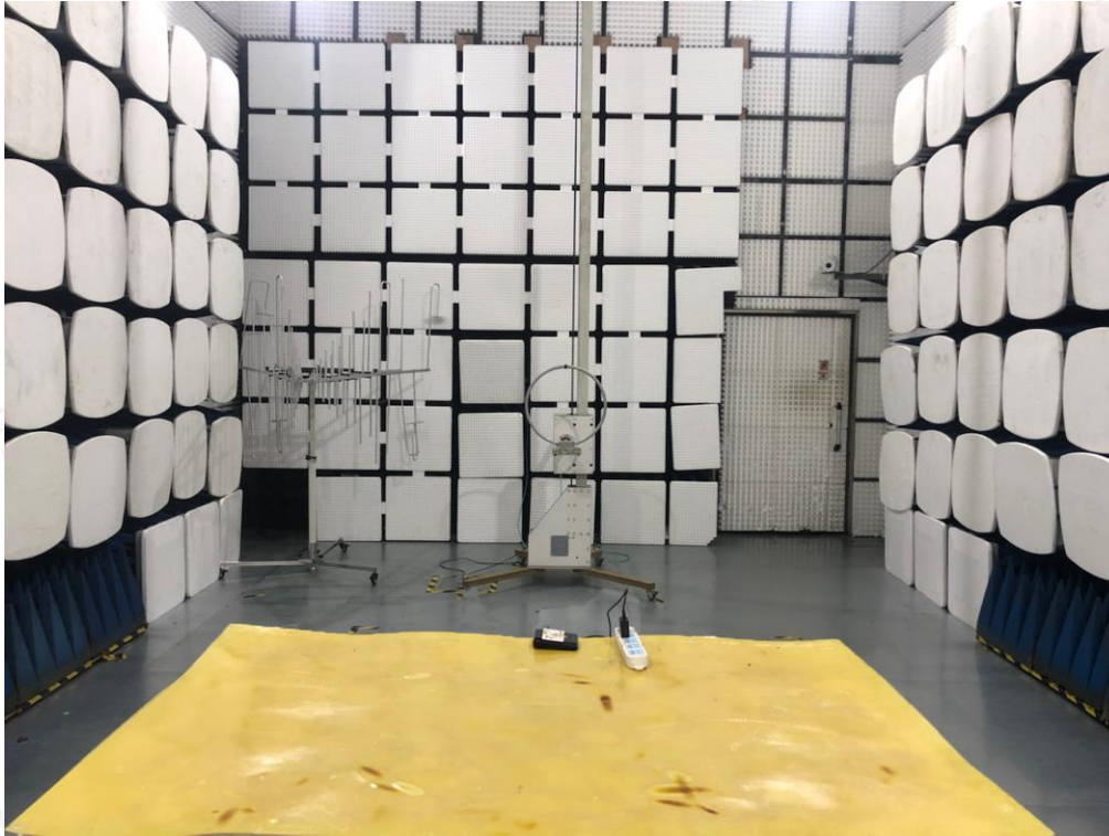
Fig. 1 (Below 30MHz)
