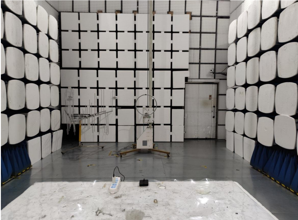
Fig. 1 (Below 30MHz)
