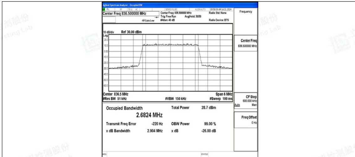
26(824-849)-3MHz-16QAM-26915-15RB#0-PASS
