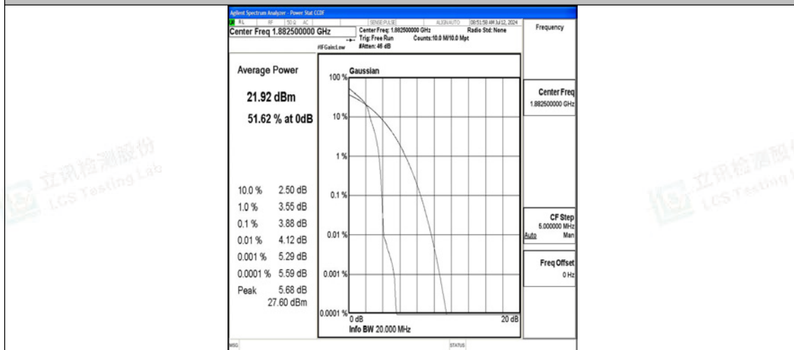
Band25-20MHz-16QAM-26365-1RB#0-PASS
