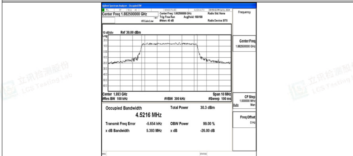
Band25-5MHz-QPSK-26365-25RB#0-PASS
