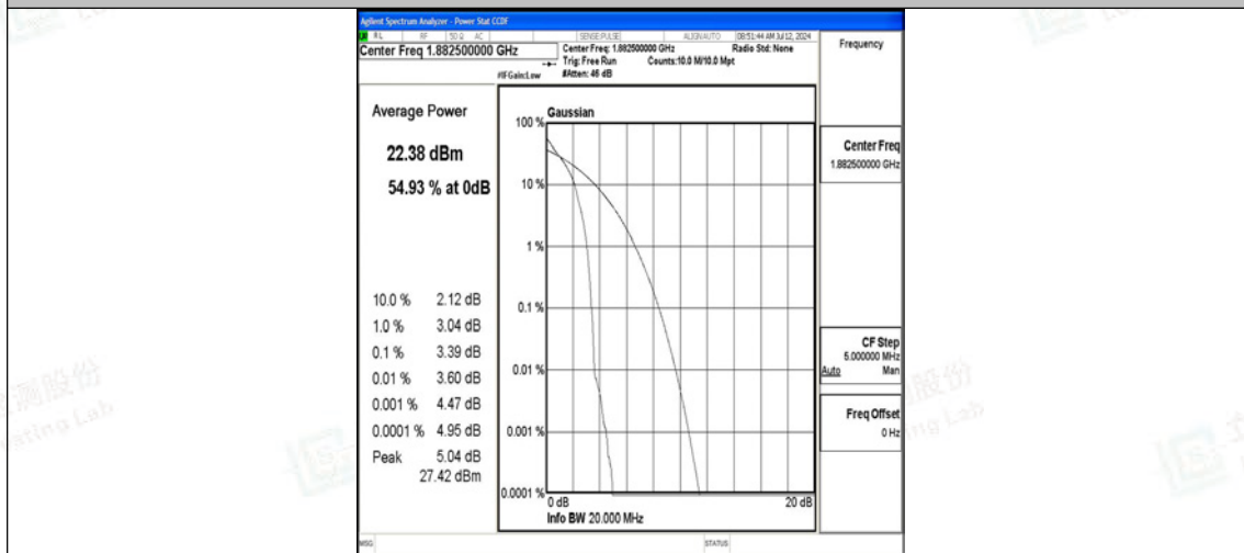
Band25-20MHz-QPSK-26365-1RB#0-PASS
