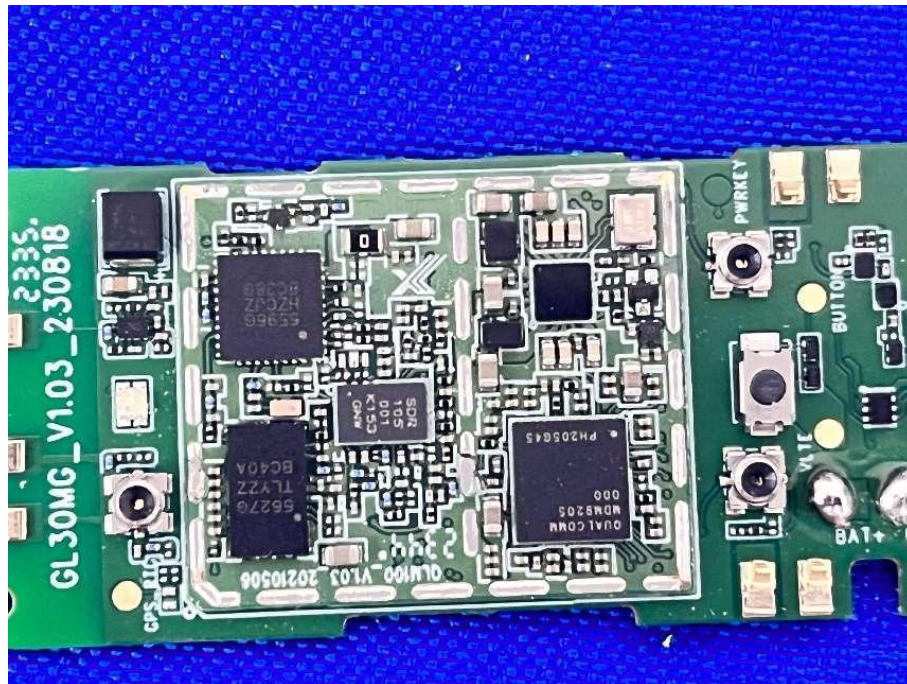
WWAN IC
