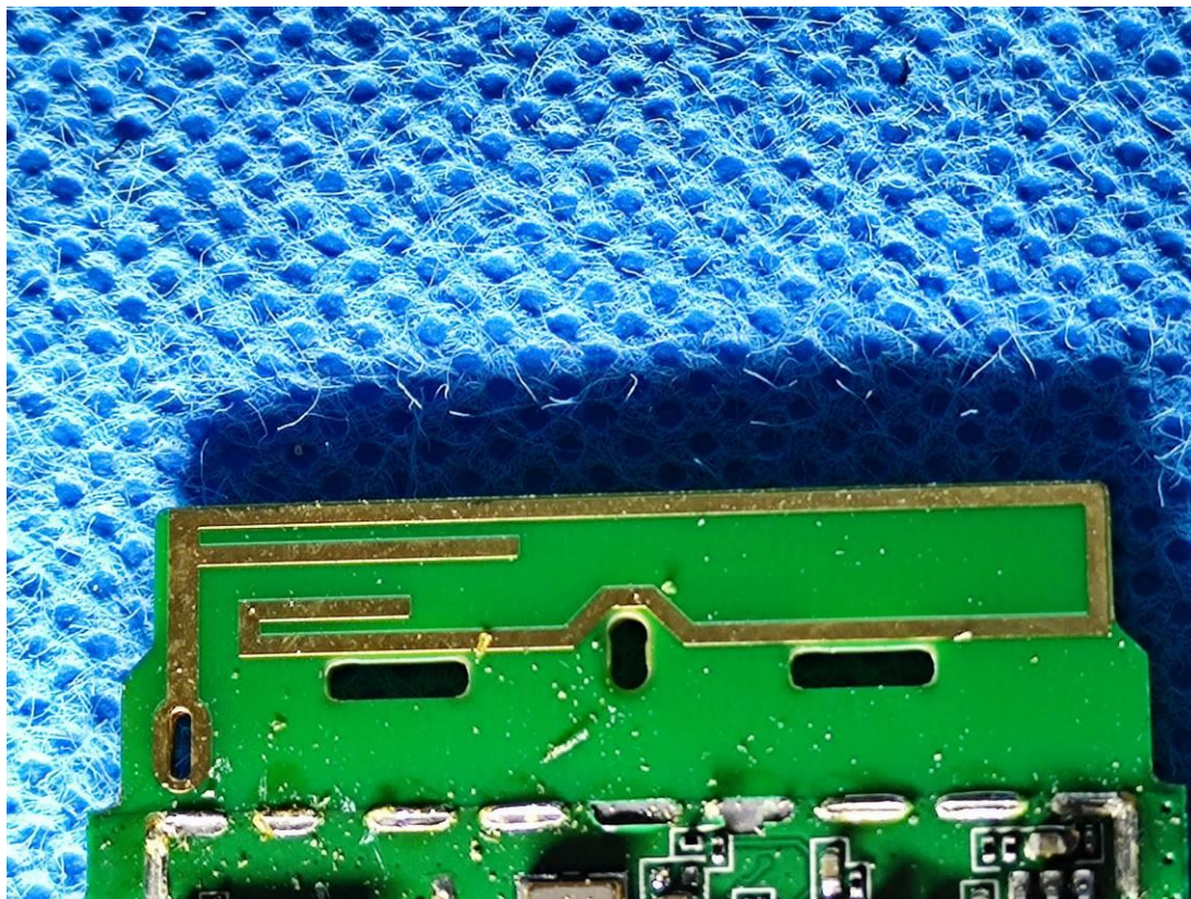
GSM Antenna
