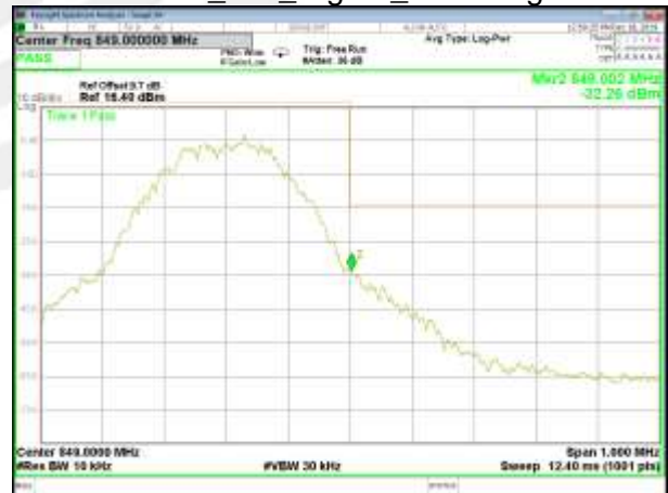
EGPRS_850_Higher_Band edge
