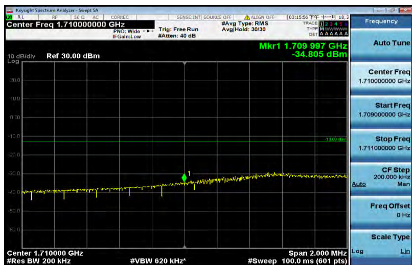
Band4-10MHz-QPSK-20000-50RB#0
