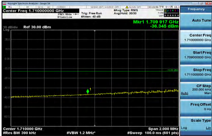
Band4-20MHz-QPSK-20050-1RB#0
