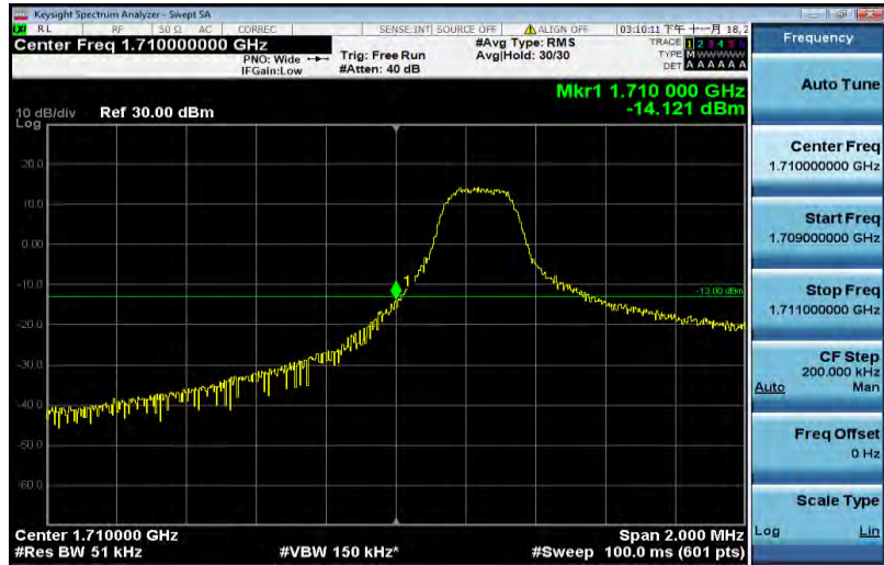
Band4-3MHz-QPSK-19965-1RB#14
