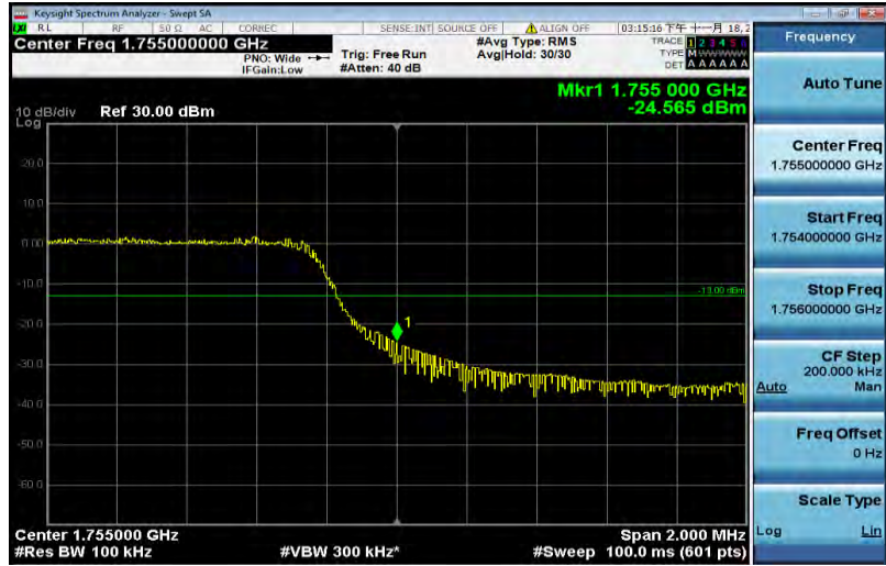
Band4-10MHz-QPSK-20000-1RB#0
