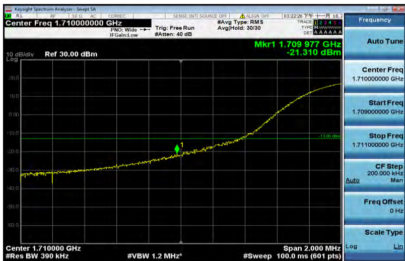
Band4-20MHz-QPSK-20050-100RB#0
