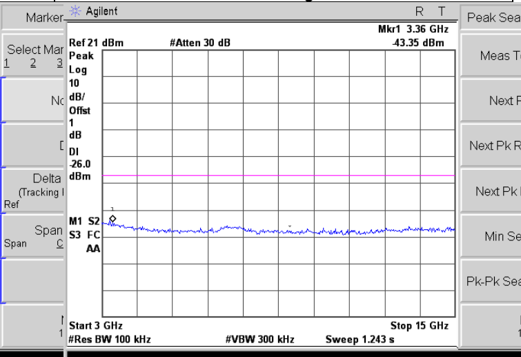
3GHz~15GHz
