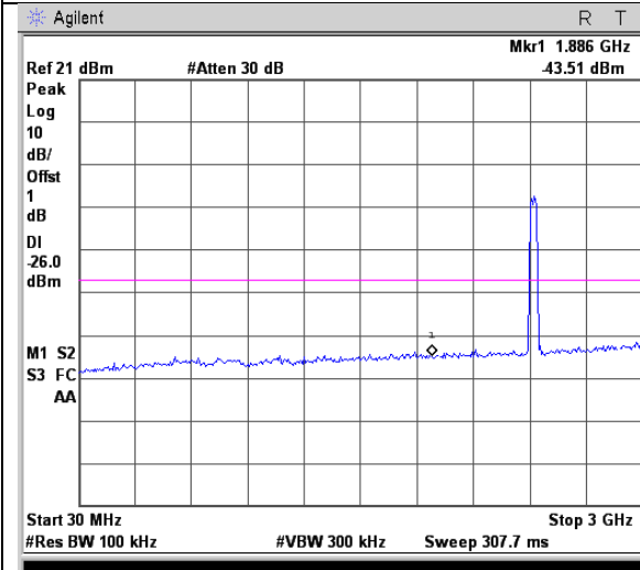
30MHz~3GHz
