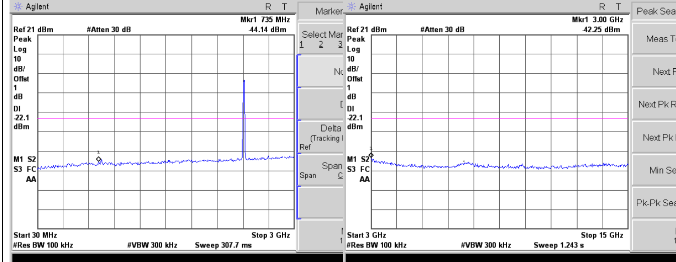
30MHz~3GHz
