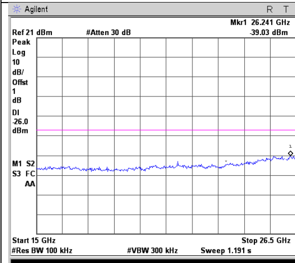
15GHz~26.5GHz
