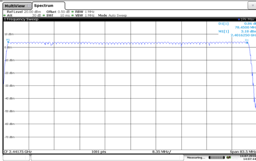
8DPSK
