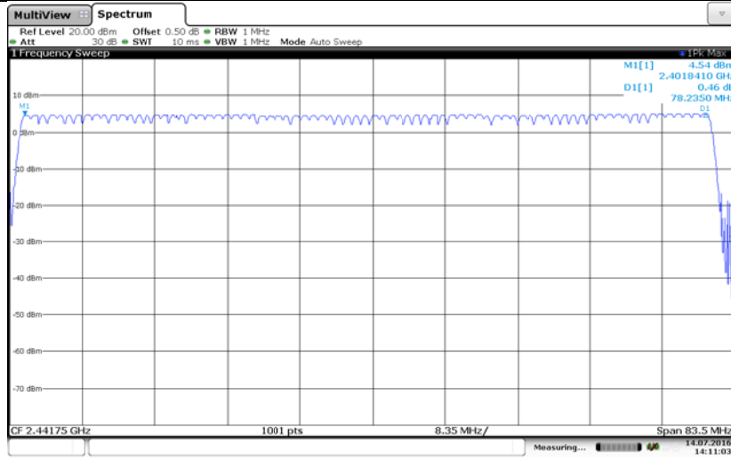
GFSK
