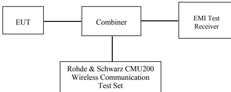
GSM/WCDMA
