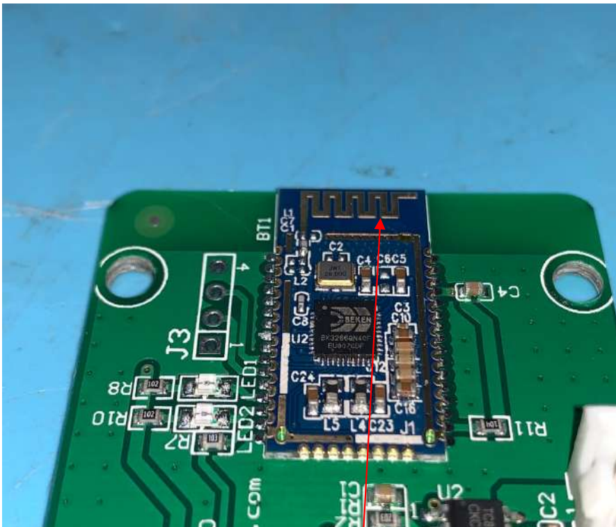
Antenna
