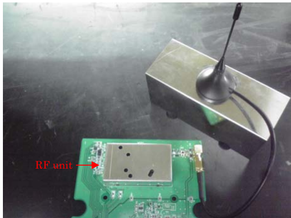
《antenna part》
