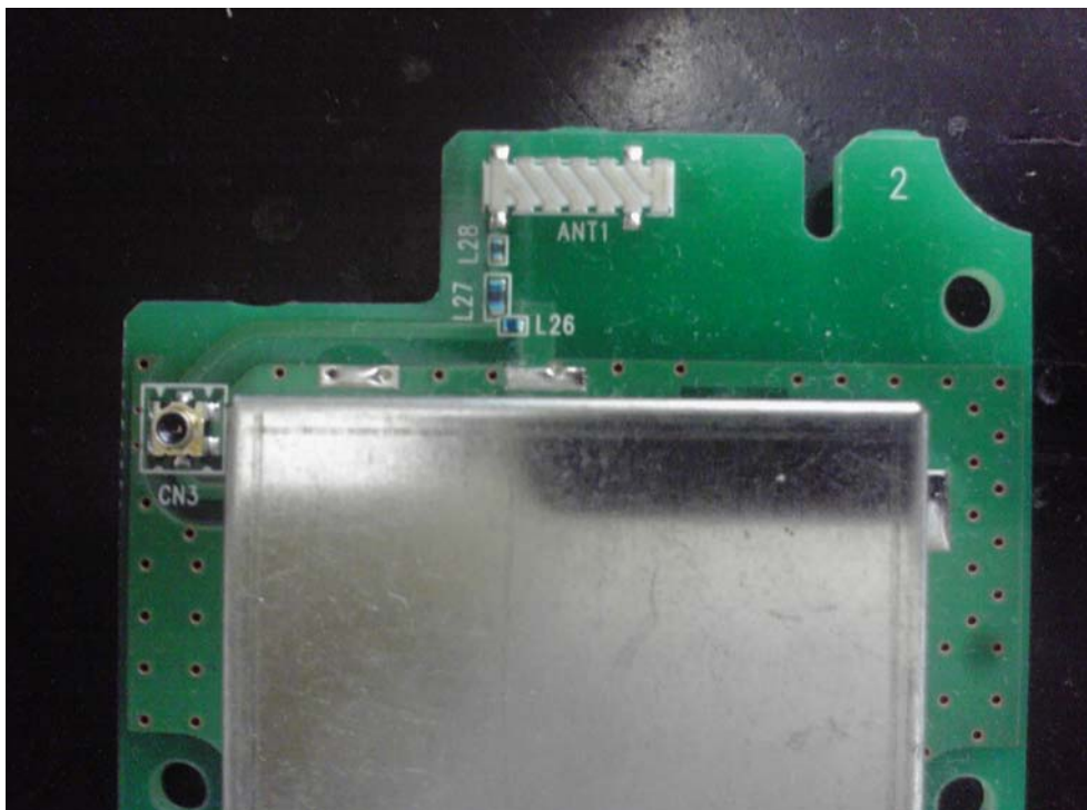
《antenna part》
