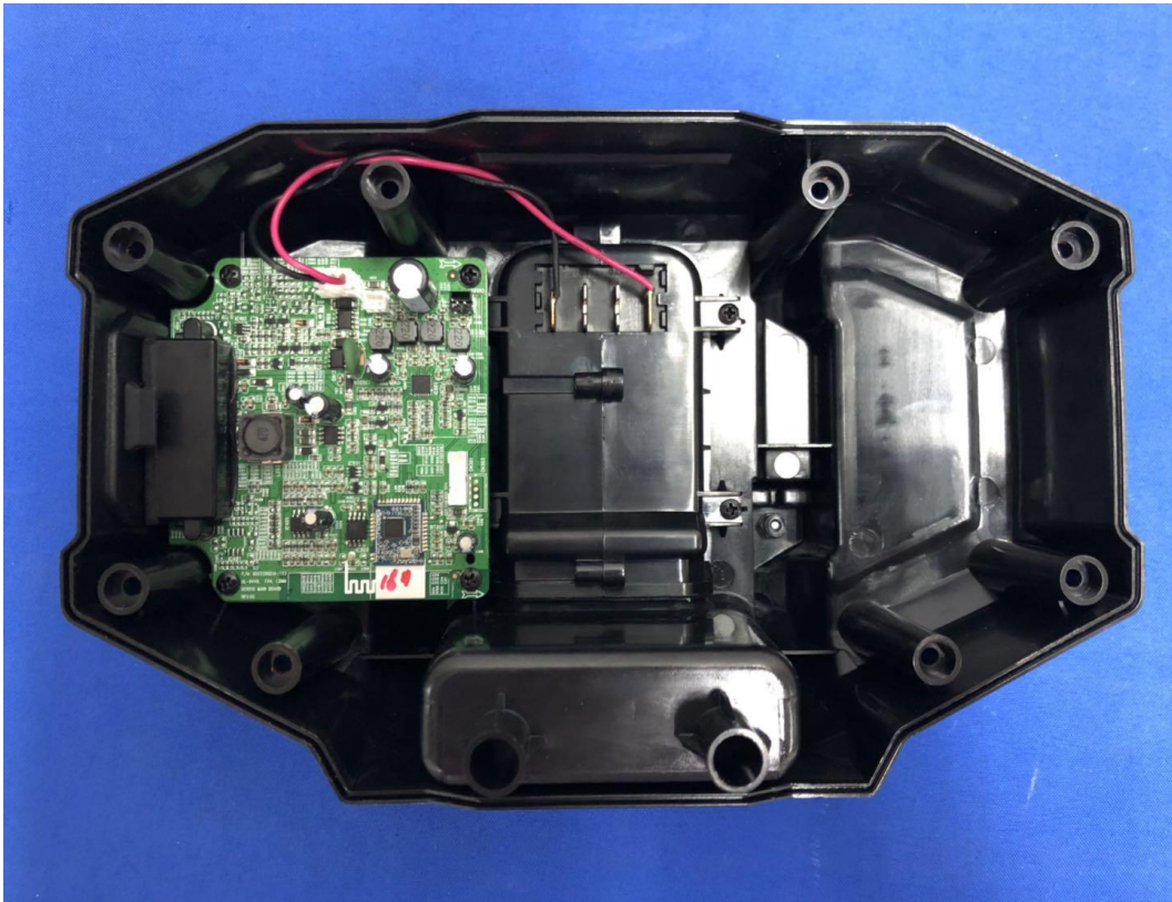
(3) EUT Photo
