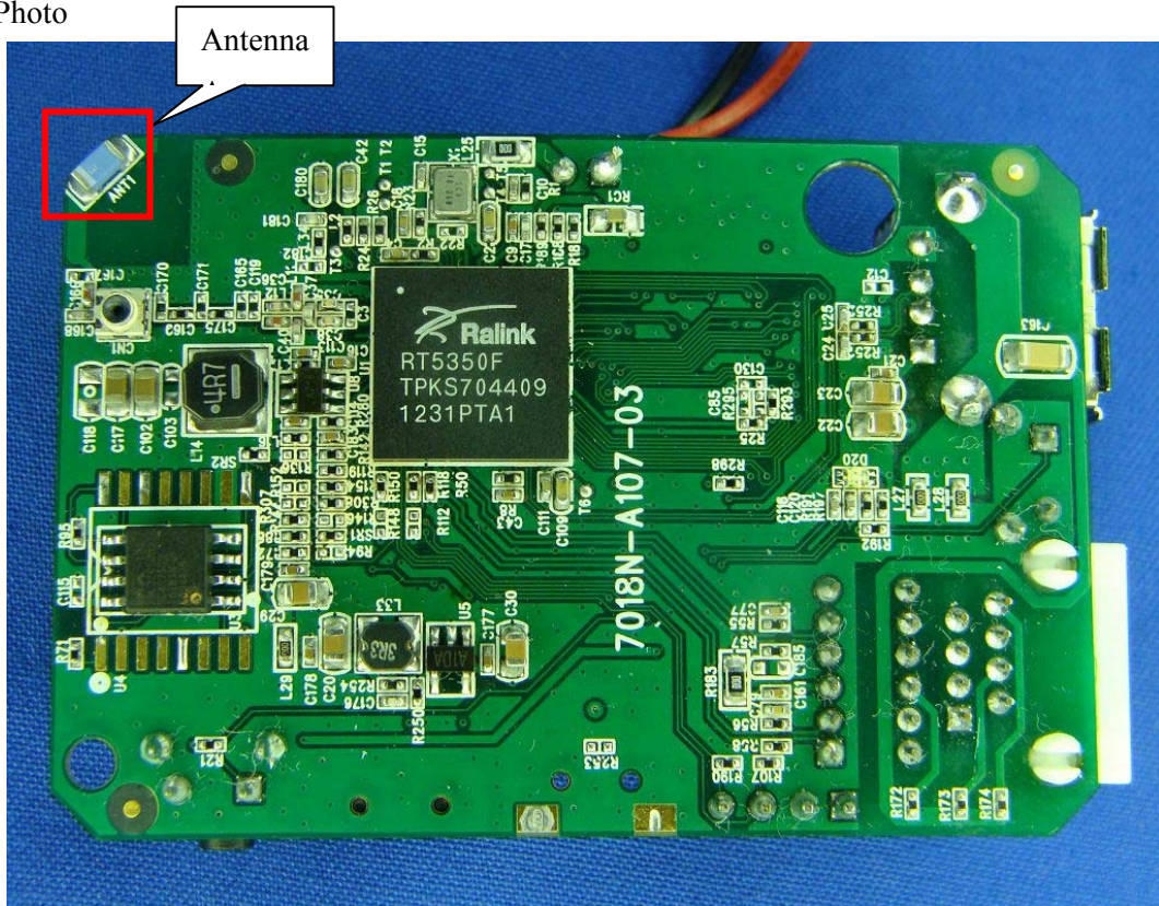
(36) EUT Photo
