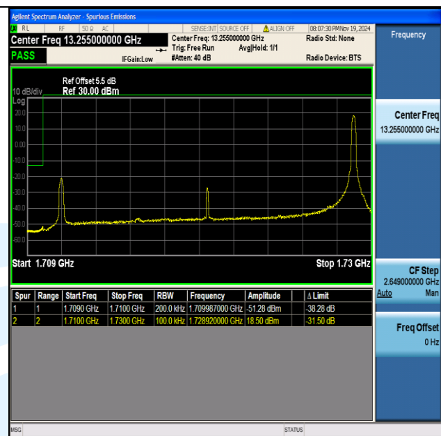
Band4 20MHz QPSK 20050 1RB#99
