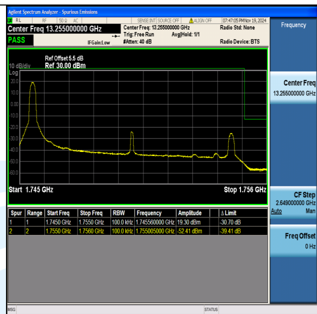
Band4 10MHz 16QAM 20350 1RB#0
