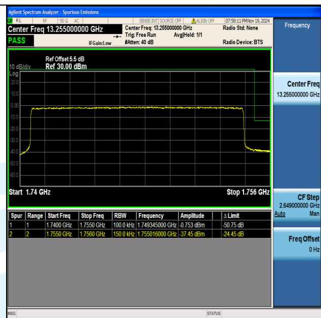
Band4 15MHz QPSK 20325 75RB#0
