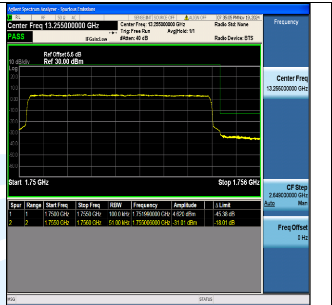
Band4 5MHz QPSK 20375 25RB#0
