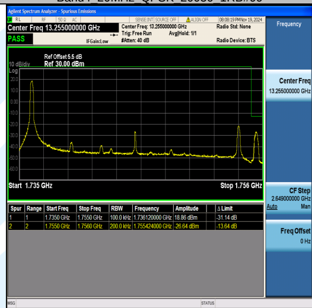
Band4 20MHz QPSK 20300 1RB#0
