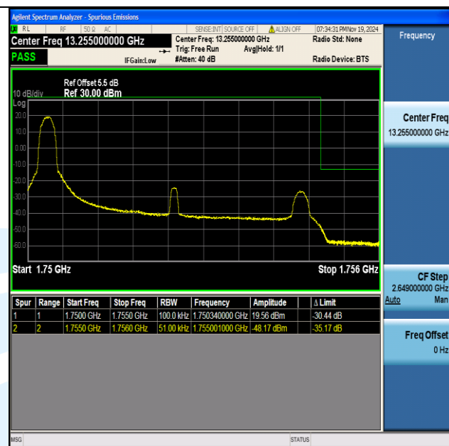
Band4 5MHz 16QAM 20375 1RB#0
