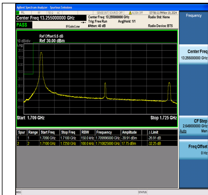
Band4 15MHz QPSK 20025 1RB#0
