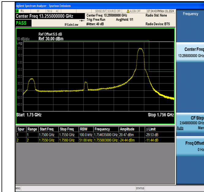
Band4 5MHz QPSK 20375 1RB#24
