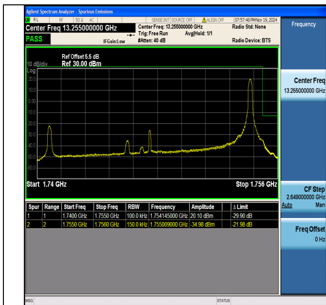
Band4 15MHz QPSK 20325 1RB#74
