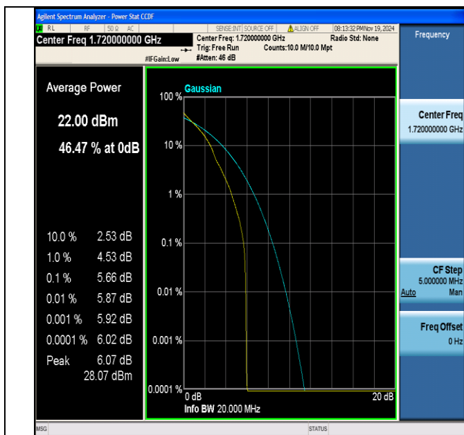
Band4-20MHz-QPSK-20050-1RB#0-PASS
