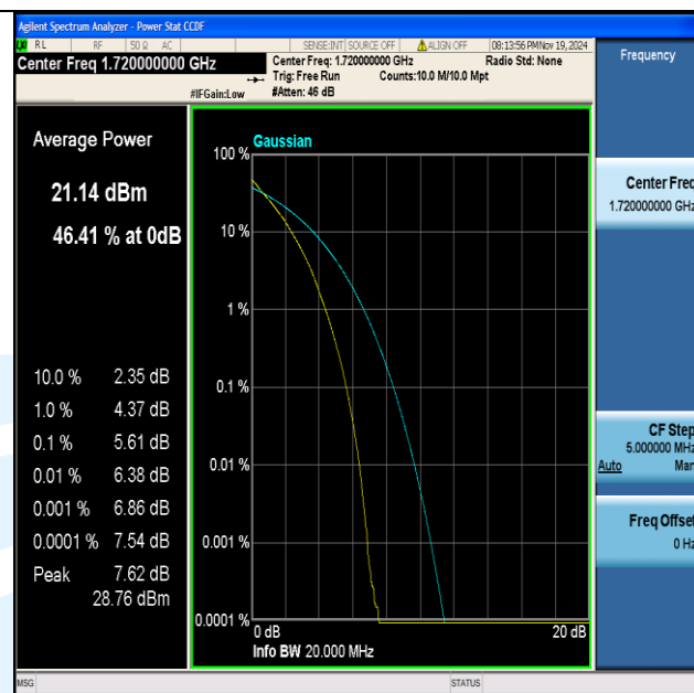
Band4-20MHz-QPSK-20050-100RB#0-PASS
