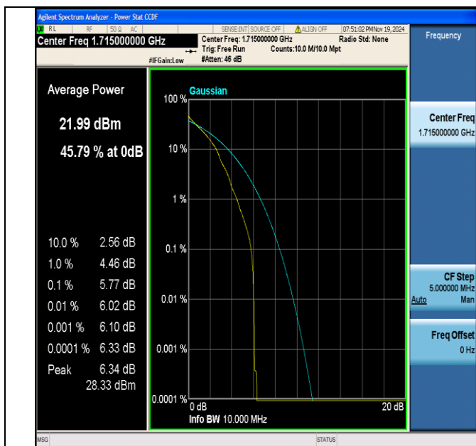
Band4-10MHz-QPSK-20000-1RB#0-PASS
