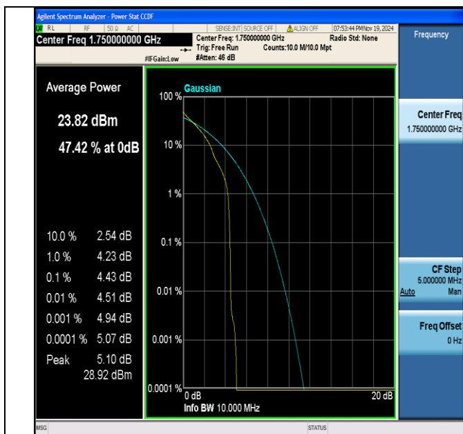
Band4-10MHz-QPSK-20350-1RB#0-PASS
