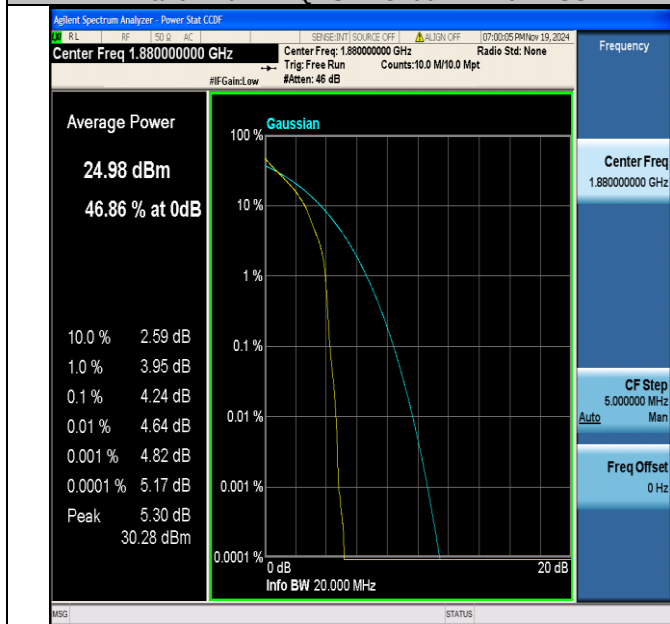
Band2-20MHz-QPSK-18900-1RB#0-PASS
