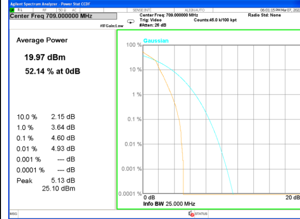
Band 17_1_Q16_Low
