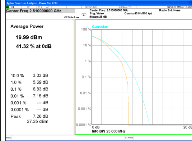
Band 7_1_Q16_Low
