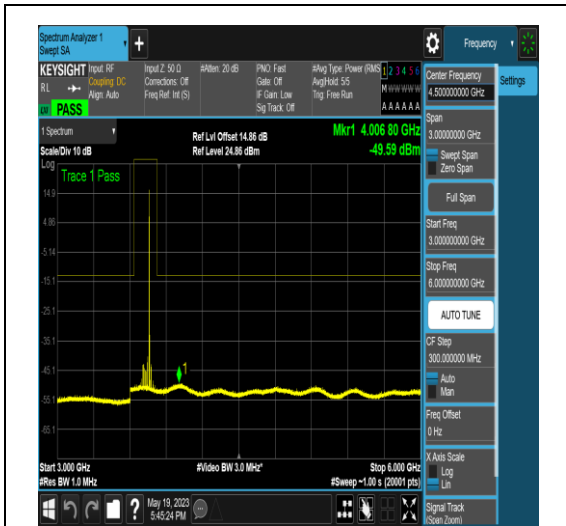
NTNV_N77-3700-3980_PC2_30_60_L_TID5_NS_01_3000_6000_#1
