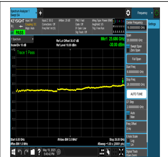
NTNV_N77-3700-3980_PC2_30_60_L_TID5_NS_01_6000_26000_#1
