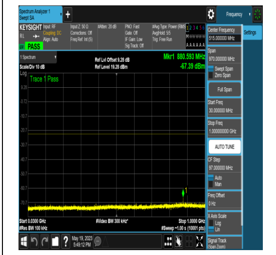
NTNV_N77-3700-3980_PC2_30_60_L_TID16_NS _01_30_1000_#1
