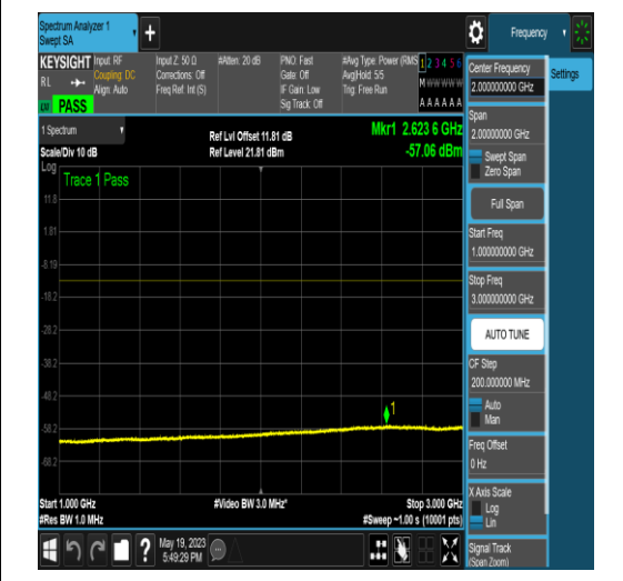
NTNV_N77-3700-3980_PC2_30_60_L_TID16_NS _01_1000_3000_#1
