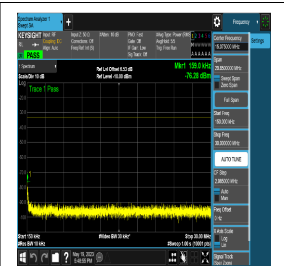
NTNV_N77-3700-3980_PC2_30_60_L_TID16_NS _01_0.15_30_#1
