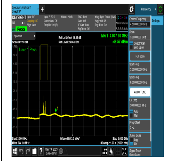
NTNV_N77-3700-3980_PC2_30_60_L_TID16_NS _01_30_1000_#1
