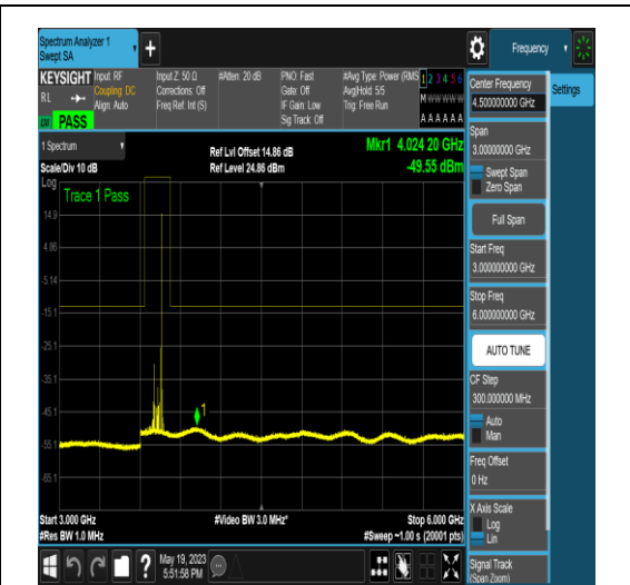
NTNV_N77-3700-3980_PC2_30_60_L_TID17_NS _01_3000_6000_#1
