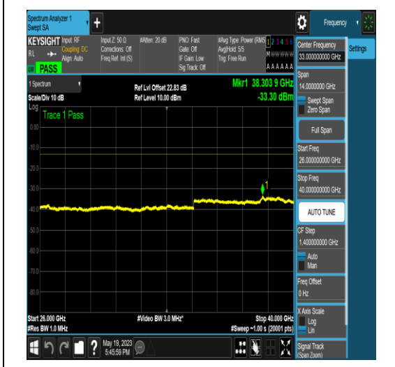
NTNV_N77-3700-3980_PC2_30_60_L_TID5_NS_01_26000_40000_#1
