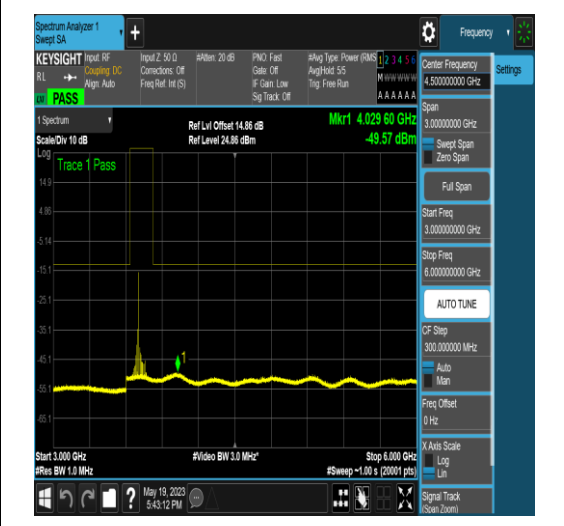
NTNV_N77-3700-3980_PC2_30_60_L_TID4_NS_01_3000_6000_#1
