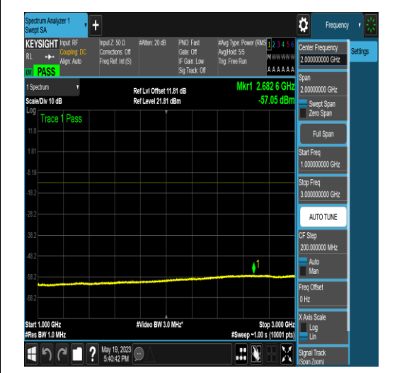
NTNV_N77-3700-3980_PC2_30_60_L_TID6_NS_01_0.15_30_#1
