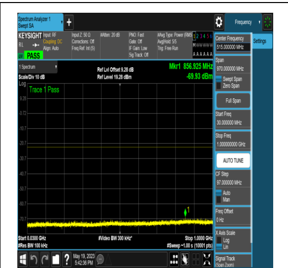
NTNV_N77-3700-3980_PC2_30_60_L_TID4_NS_01_30_1000_#1
