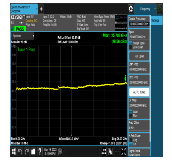
NTNV_N77-3700-3980_PC2_30_50_M_TID6_NS _01_6000_26000_#1
