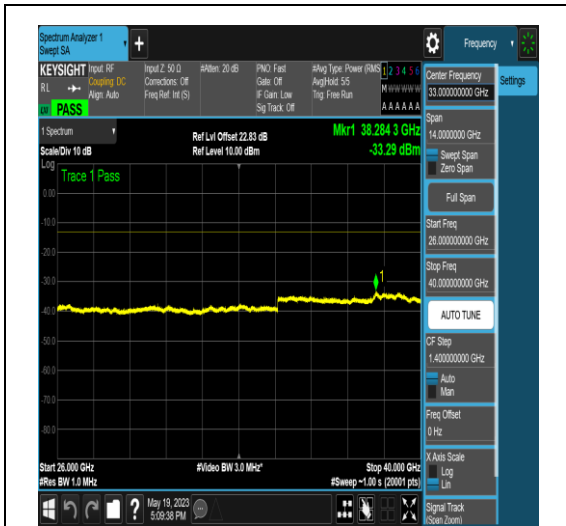
NTNV_N77-3700-3980_PC2_30_50_L_TID16_NS _01_26000_40000_#1
