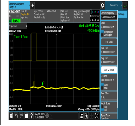
NTNV_N77-3700-3980_PC2_30_50_L_TID5_NS_01_30_1000_#1
