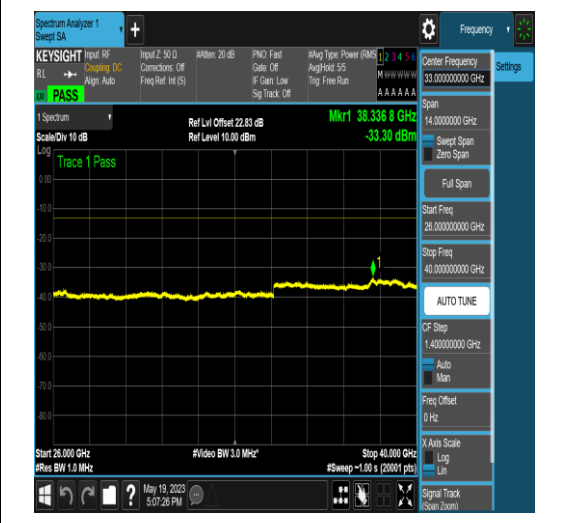
NTNV_N77-3700-3980_PC2_30_50_L_TID18_NS _01_26000_40000_#1
