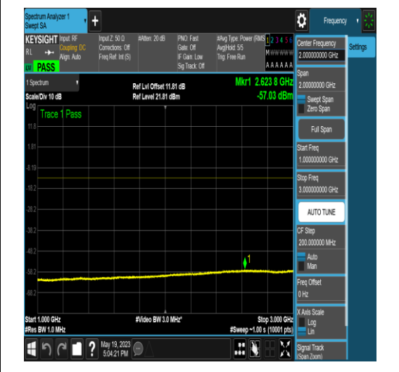
NTNV_N77-3700-3980_PC2_30_50_L_TID5_NS_01_1000_3000_#1
