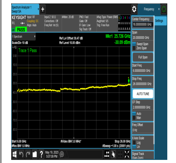
NTNV_N77-3700-3980_PC2_30_50_L_TID18_NS _01_6000_26000_#1
