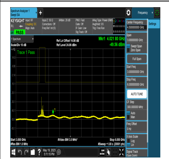
NTNV_N77-3700-3980_PC2_30_50_L_TID17_NS _01_30_1000_#1
