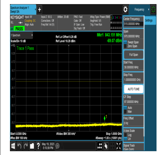
NTNV_N77-3700-3980_PC2_30_50_L_TID17_NS _01_30_1000_#1
