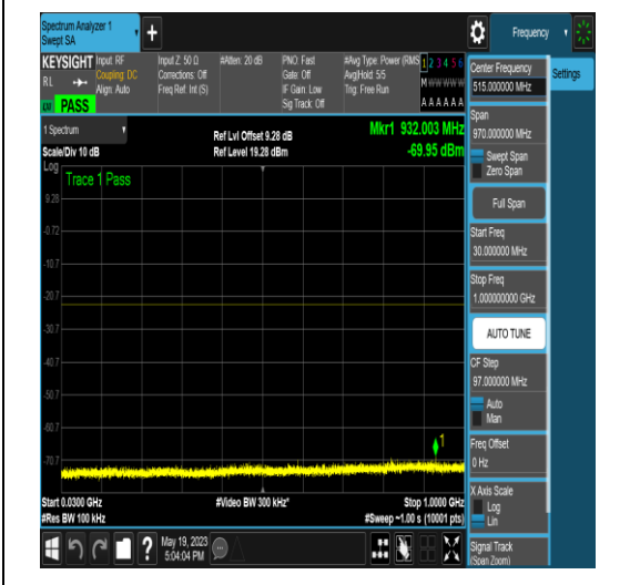
NTNV_N77-3700-3980_PC2_30_50_L_TID5_NS_01_30_1000_#1
