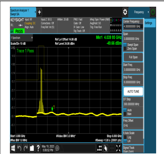
NTNV_N77-3700-3980_PC2_30_50_L_TID18_NS _01_3000_6000_#1
