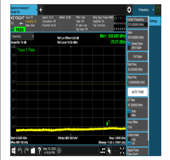
NTNV_N77-3700-3980_PC2_30_40_L_TID18_NS_01_30_1000_#1
