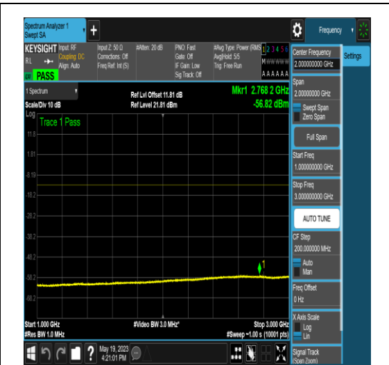
NTNV_N77-3700-3980_PC2_30_40_L_TID16_NS _01_1000_3000_#1
