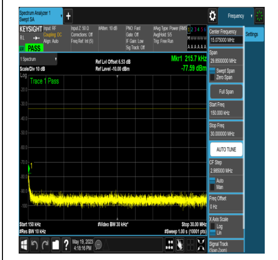
NTNV_N77-3700-3980_PC2_30_40_L_TID18_NS_01_0.15_30_#1
