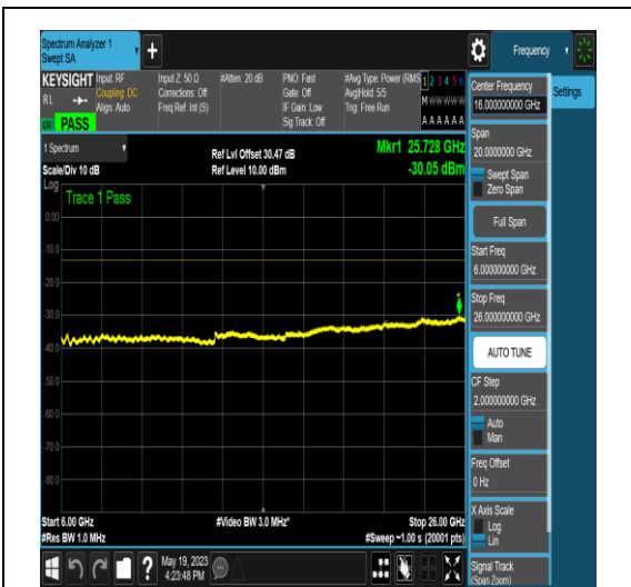
NTNV_N77-3700-3980_PC2_30_40_L_TID17_NS _01_6000_26000_#1
