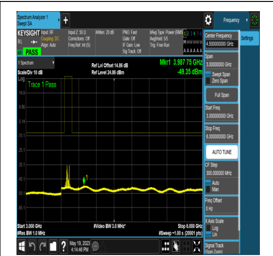
NTNV_N77-3700-3980_PC2_30_40_L_TID4_NS_01_3000_6000_#1
