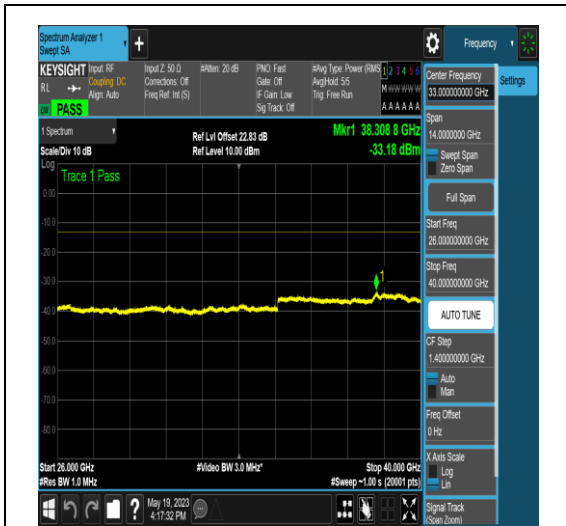
NTNV_N77-3700-3980_PC2_30_40_L_TID5_NS_01_26000_40000_#1
