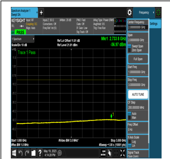
NTNV_N77-3700-3980_PC2_30_40_L_TID4_NS_01_1000_3000_#1
