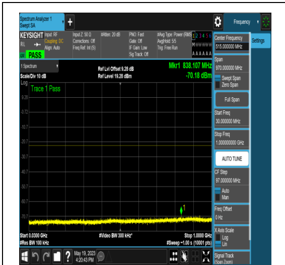
NTNV_N77-3700-3980_PC2_30_40_L_TID16_NS _01_30_1000_#1
