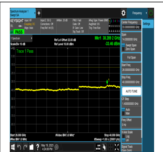
NTNV_N77-3700-3980_PC2_30_40_L_TID17_NS _01_26000_40000_#1
