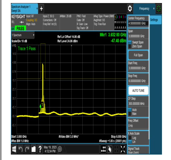
NTNV_N77-3700-3980_PC2_30_40_L_TID6_NS_01_30_1000_#1
