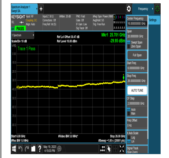
NTNV_N77-3700-3980_PC2_30_40_L_TID4_NS_01_6000_26000_#1
