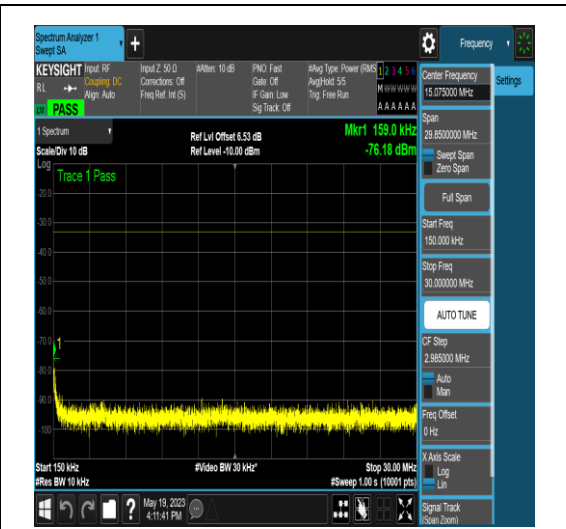
NTNV_N77-3700-3980_PC2_30_40_L_TID6_NS_01_0.15_30_#1
