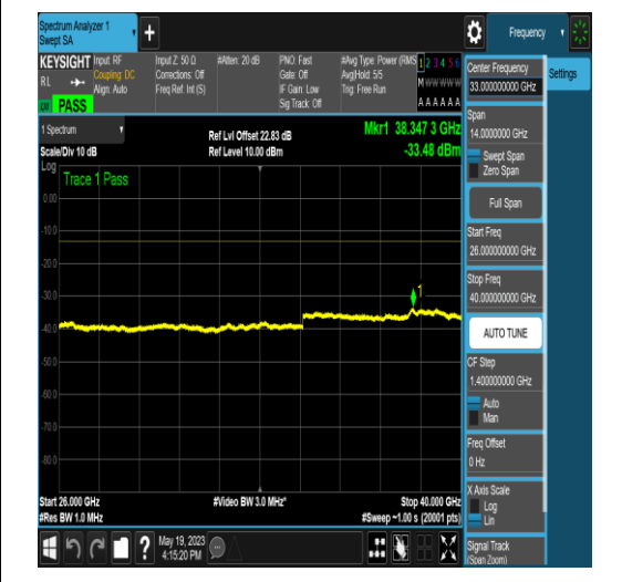
NTNV_N77-3700-3980_PC2_30_40_L_TID4_NS_01_26000_40000_#1
