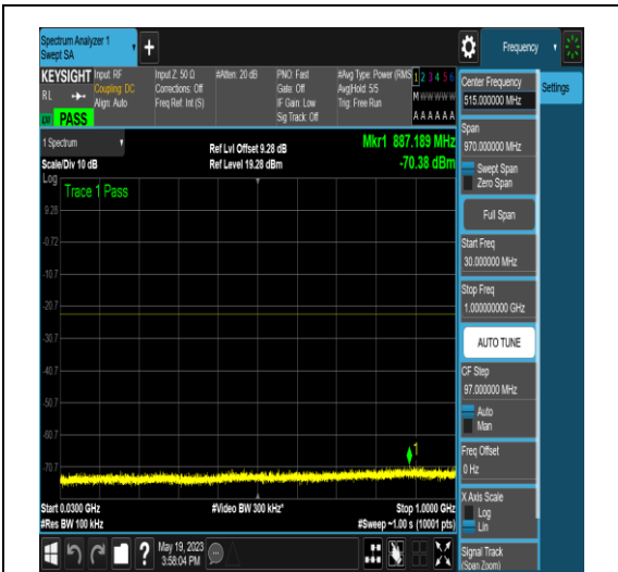
NTNV_N77-3700-3980_PC2_30_20_H_TID6_NS _01_30_1000_#1
