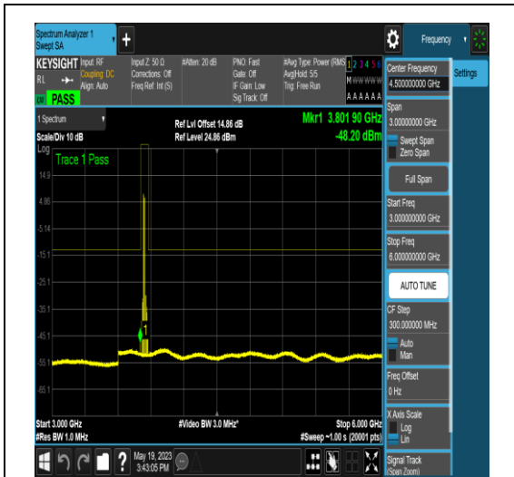
NTNV_N77-3700-3980_PC2_30_20_M_TID6_NS _01_3000_6000_#1
