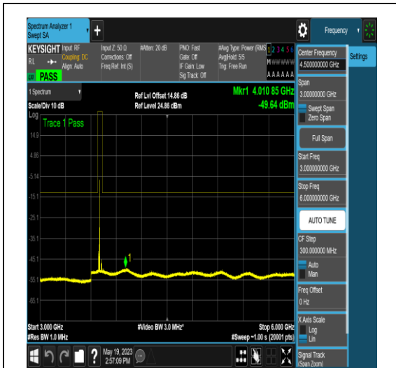
NTNV_N77-3700-3980_PC2_30_15_L_TID16_NS _01_3000_6000_#1
