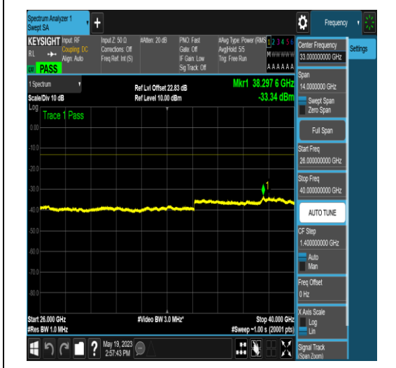
NTNV_N77-3700-3980_PC2_30_15_L_TID16_NS _01_26000_40000_#1
