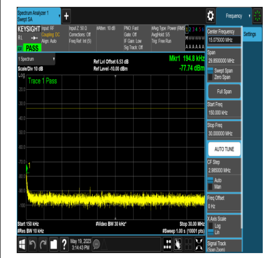
NTNV_N77-3700-3980_PC2_30_15_H_TID6_NS _01_0.15_30_#1
