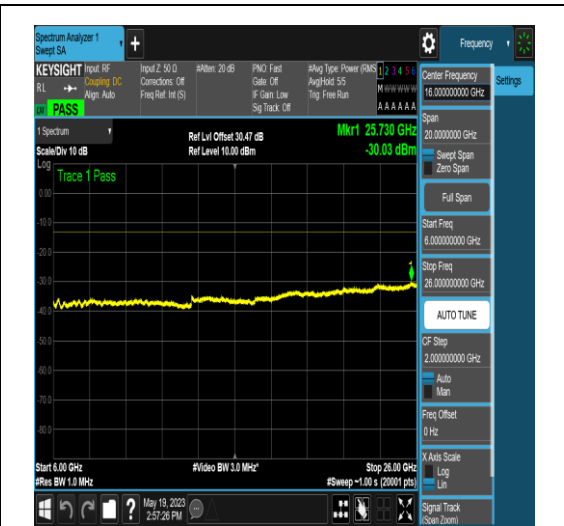
NTNV_N77-3700-3980_PC2_30_15_L_TID16_NS _01_6000_26000_#1
