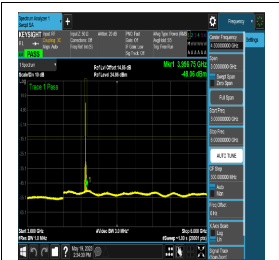
NTNV_N77-3700-3980_PC2_30_10_H_TID6_NS _01_3000_6000_#1
