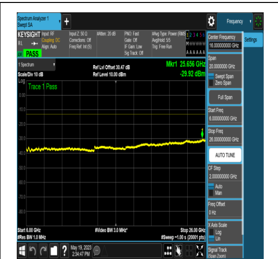
NTNV_N77-3700-3980_PC2_30_10_H_TID6_NS _01_6000_26000_#1
