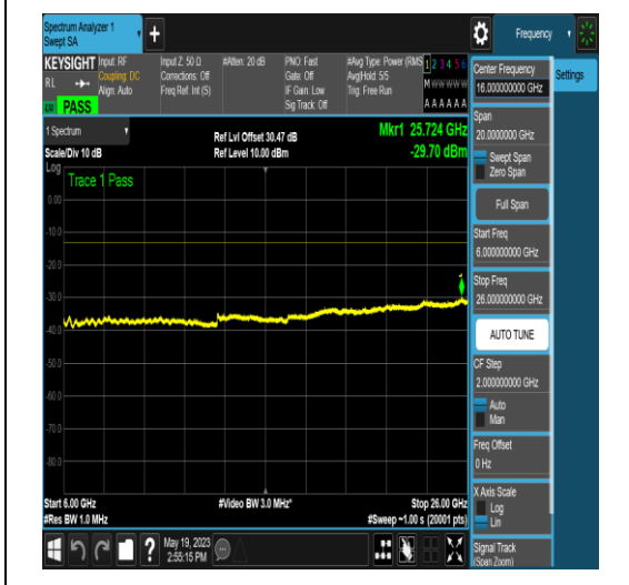
NTNV_N77-3700-3980_PC2_30_15_L_TID18_NS _01_1000_3000_#1
