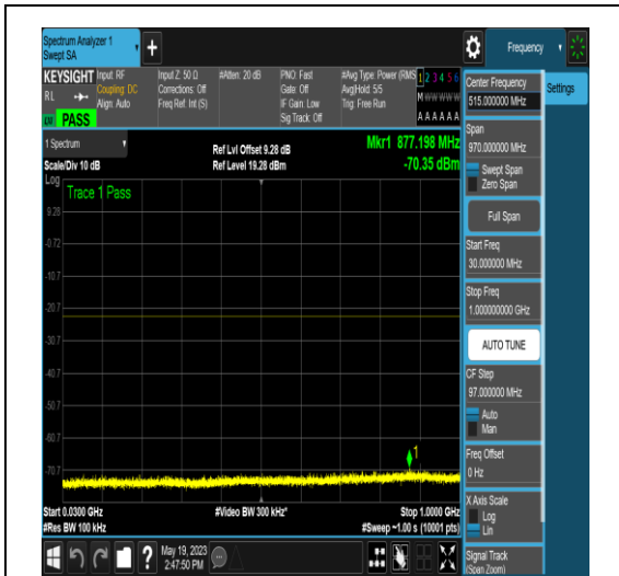
NTNV_N77-3700-3980_PC2_30_15_L_TID6_NS_01_30_1000_#1
