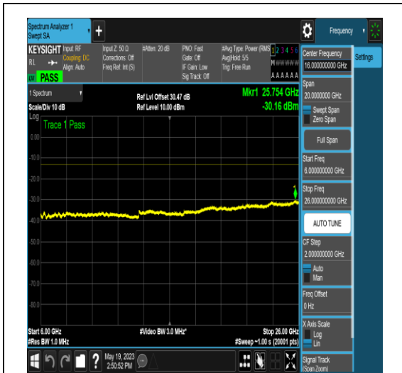
NTNV_N77-3700-3980_PC2_30_15_L_TID4_NS_01_6000_26000_#1
