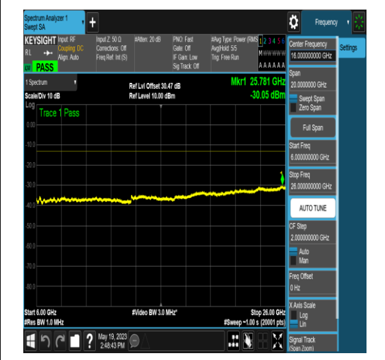
NTNV_N77-3700-3980_PC2_30_15_L_TID6_NS_01_6000_26000_#1
