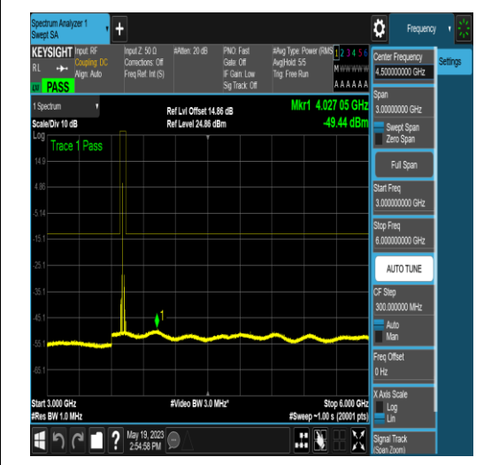
NTNV_N77-3700-3980_PC2_30_15_L_TID18_NS _01_3000_6000_#1
