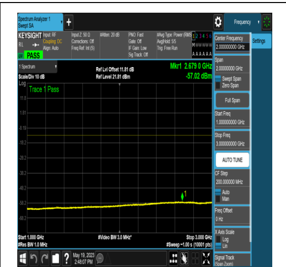
NTNV_N77-3700-3980_PC2_30_15_L_TID6_NS_01_1000_3000_#1
