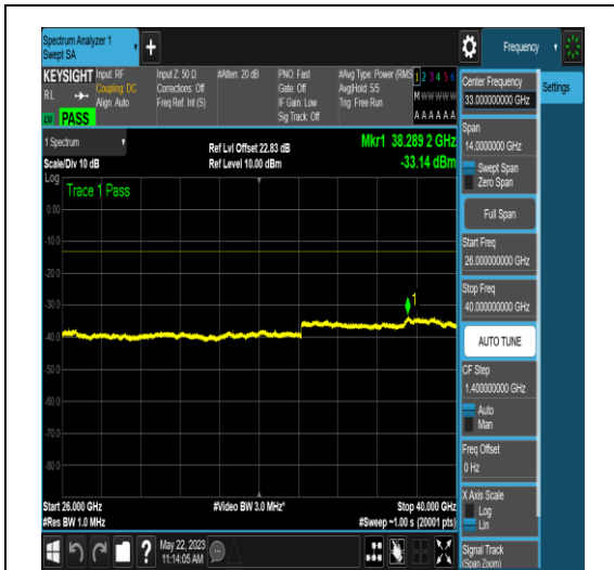
NTNV_N77-3700-3980_PC2_30_90_L_TID6_NS_01_26000_40000_#1
