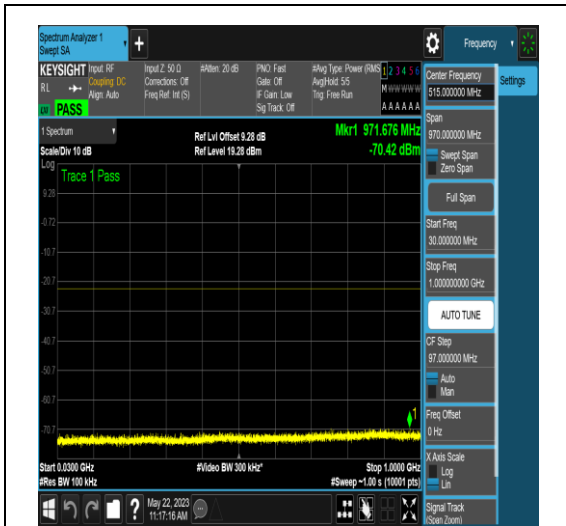
NTNV_N77-3700-3980_PC2_30_90_L_TID5_NS_01_30_1000_#1
