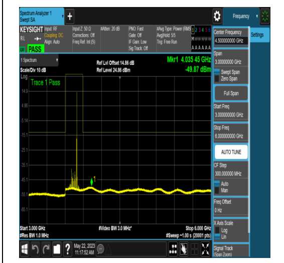
NTNV_N77-3700-3980_PC2_30_90_L_TID5_NS_01_3000_6000_#1
