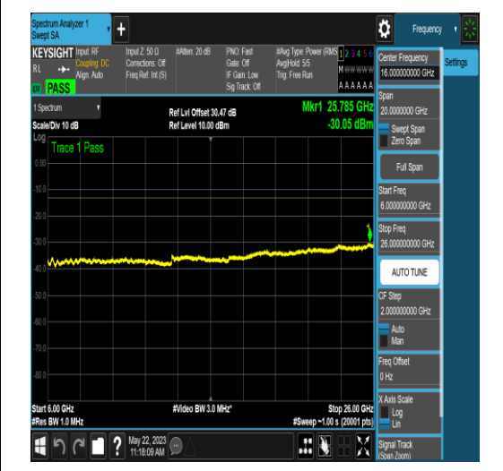
NTNV_N77-3700-3980_PC2_30_90_L_TID5_NS_01_6000_26000_#1
