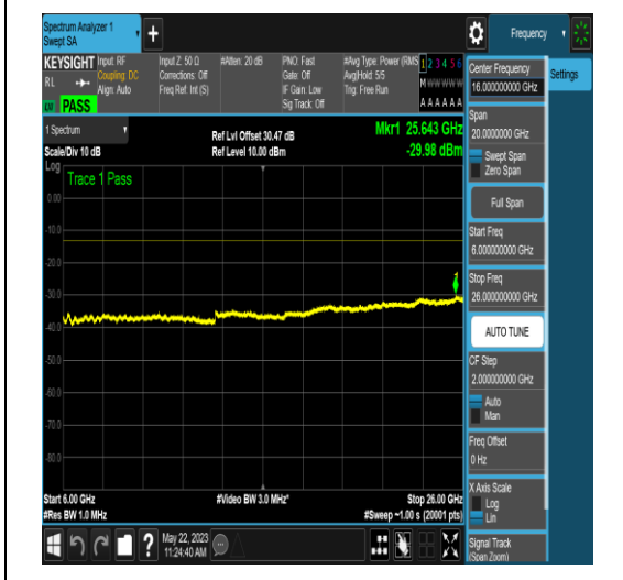
NTNV_N77-3700-3980_PC2_30_90_L_TID17_NS _01_1000_3000_#1
