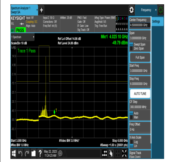
NTNV_N77-3700-3980_PC2_30_90_L_TID17_NS _01_3000_6000_#1
