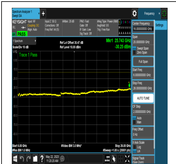
NTNV_N77-3700-3980_PC2_30_90_L_TID18_NS _01_6000_26000_#1
