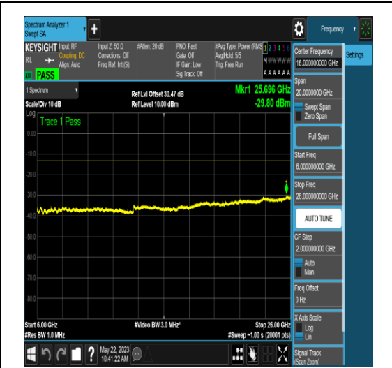
NTNV_N77-3700-3980_PC2_30_80_L_TID16_NS _01_6000_26000_#1
