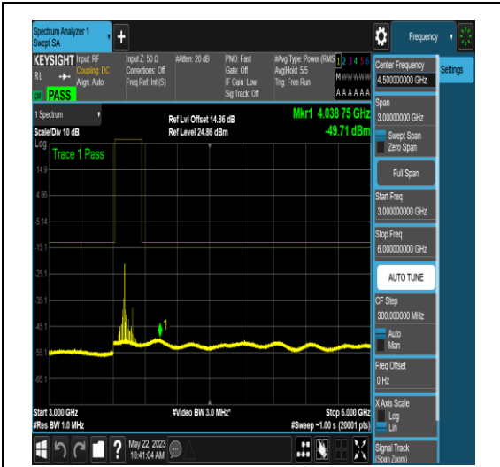
NTNV_N77-3700-3980_PC2_30_80_L_TID16_NS _01_3000_6000_#1
