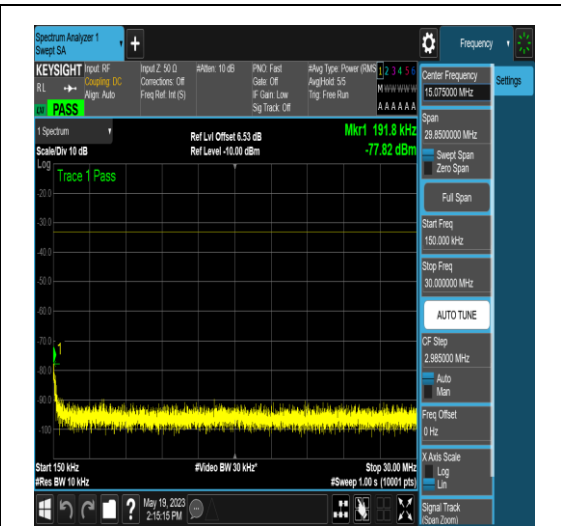
NTNV_N77-3700-3980_PC2_30_10_L_TID16_NS _01_0.15_30_#1
