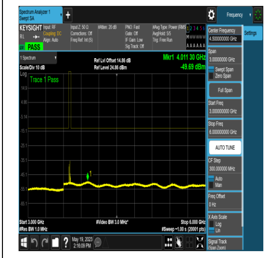
NTNV_N77-3700-3980_PC2_30_10_L_TID16_NS _01_30_1000_#1
