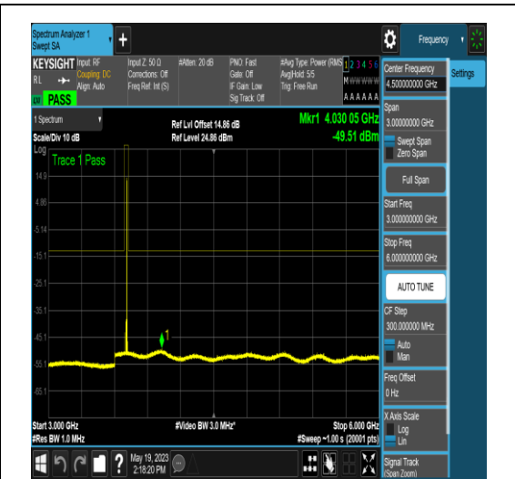
NTNV_N77-3700-3980_PC2_30_10_L_TID17_NS _01_3000_6000_#1
