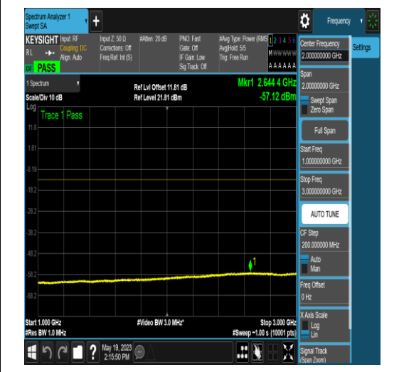
NTNV_N77-3700-3980_PC2_30_10_L_TID16_NS _01_1000_3000_#1
