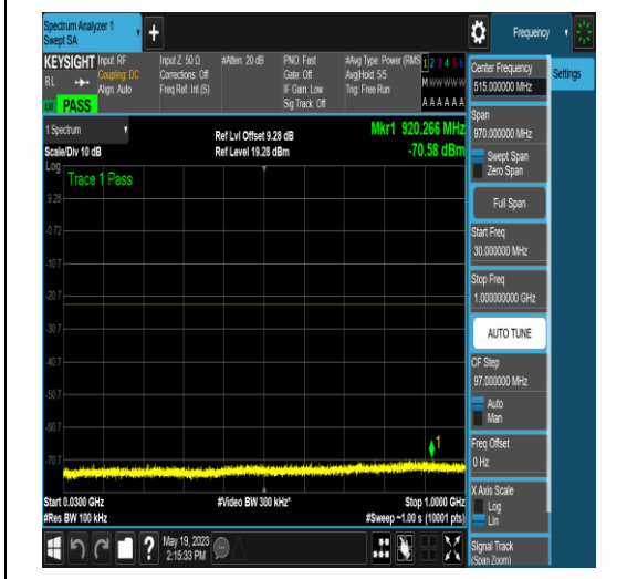
NTNV_N77-3700-3980_PC2_30_10_L_TID16_NS _01_30_1000_#1
