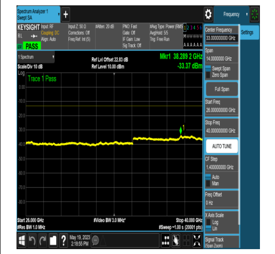
NTNV_N77-3700-3980_PC2_30_10_L_TID17_NS _01_26000_40000_#1
