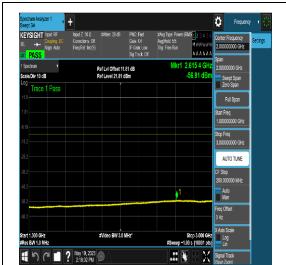
NTNV_N77-3700-3980_PC2_30_10_L_TID17_NS _01_1000_3000_#1
