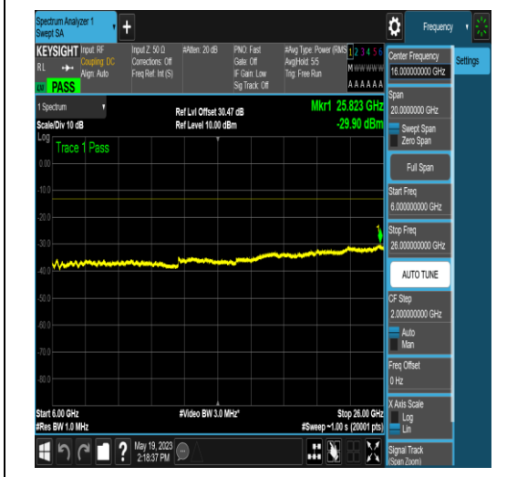
NTNV_N77-3700-3980_PC2_30_10_L_TID17_NS _01_6000_26000_#1
