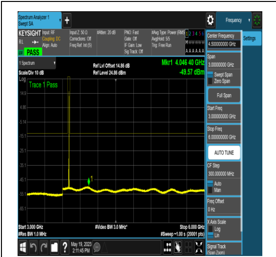
NTNV_N77-3700-3980_PC2_30_10_L_TID5_NS_01_3000_6000_#1
