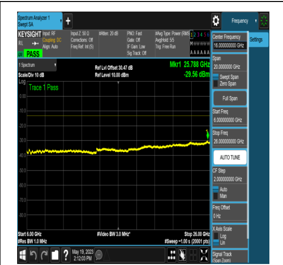
NTNV_N77-3700-3980_PC2_30_10_L_TID5_NS_01_6000_26000_#1
