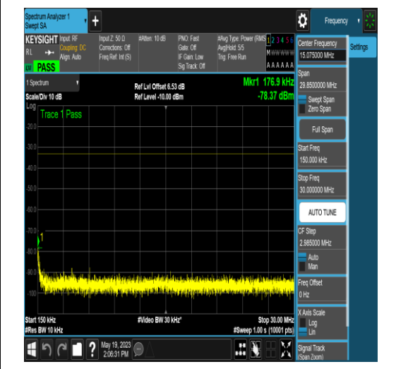
NTNV_N77-3700-3980_PC2_30_10_L_TID6_NS 01_0.15_30_#1
