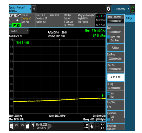
NTNV_N77-3700-3980_PC2_30_10_L_TID6_NS 01_0.15_30_#1
