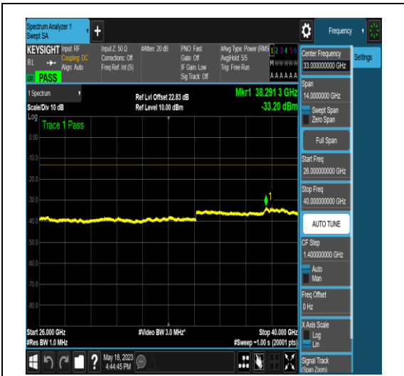
NTNV_N77-3450-3550_PC2_30_80_L_TID6_N/A _26000_40000_#1
