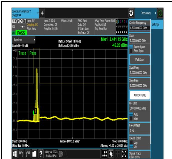
NTNV_N77-3450-3550_PC2_30_50_H_TID6_N/A _3000_6000_#1
