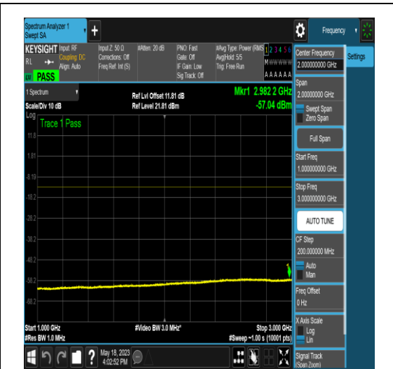
NTNV_N77-3450-3550_PC2_30_60_L_TID6_N/A _1000_3000_#1
