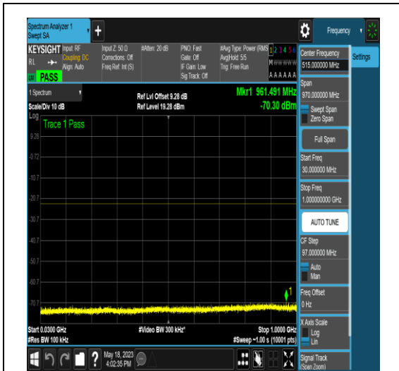
NTNV_N77-3450-3550_PC2_30_60_L_TID6_N/A _30_1000_#1
