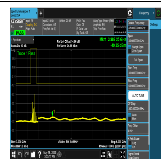
NTNV_N77-3450-3550_PC2_30_50_L_TID17_N/ A_3000_6000_#1
