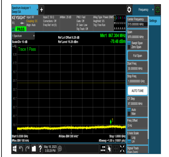
NTNV_N77-3450-3550_PC2_30_50_L_TID16_N/ A_30_1000_#1
