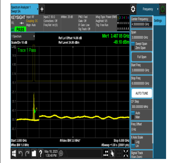
NTNV_N77-3450-3550_PC2_30_15_L_TID17_N/ A_3000_6000_#1
