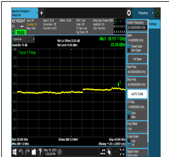
NTNV_N77-3450-3550_PC2_30_15_L_TID6_N/A _26000_40000_#1
