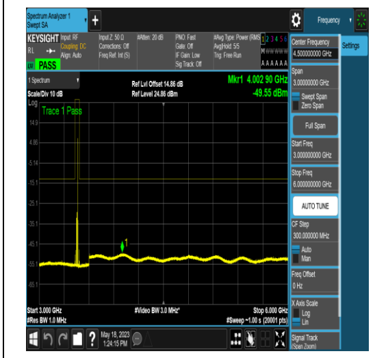
NTNV_N77-3450-3550_PC2_30_15_L_TID5_N/A _3000_6000_#1
